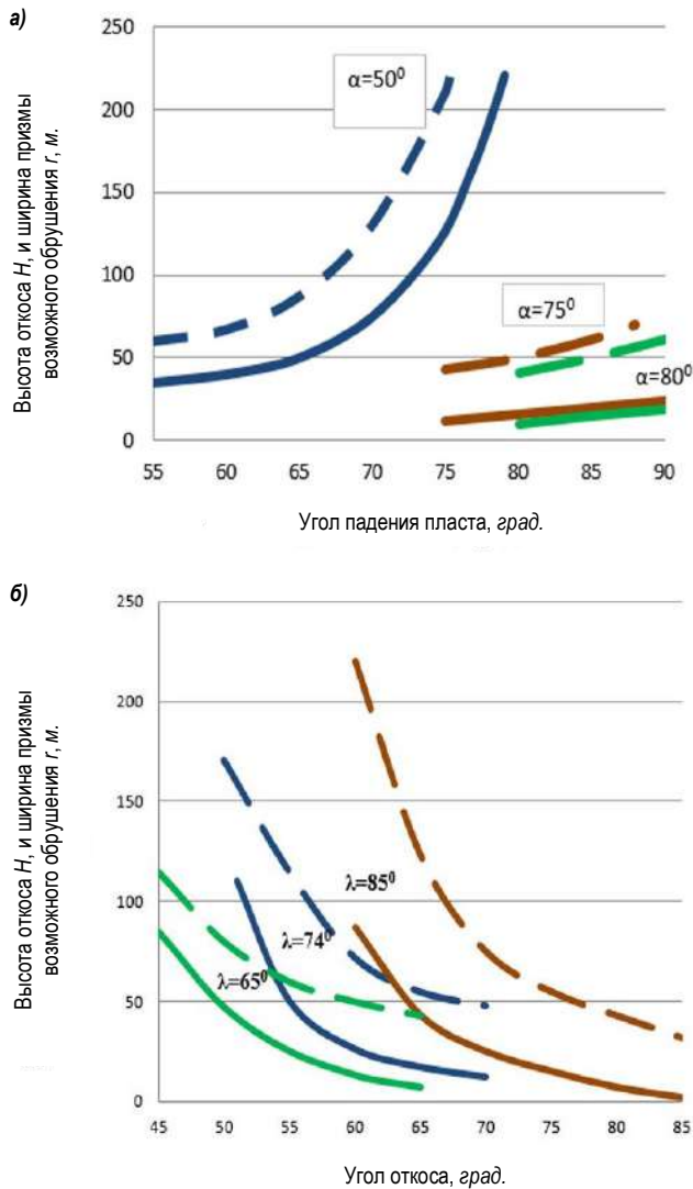
Рис. 1. Зависимости высоты откоса уступа H и ширины призмы возможного обрушения r от угла падения слоистости a при a=50, 75, 80^\circ (а) и угла откоса \lambda при \lambda=65, 74, 85^\circ (б) для массива со следующими характеристиками: C=0,2 МПа; C=0,012 МПа; j=30^\circ ; j=27^\circ
