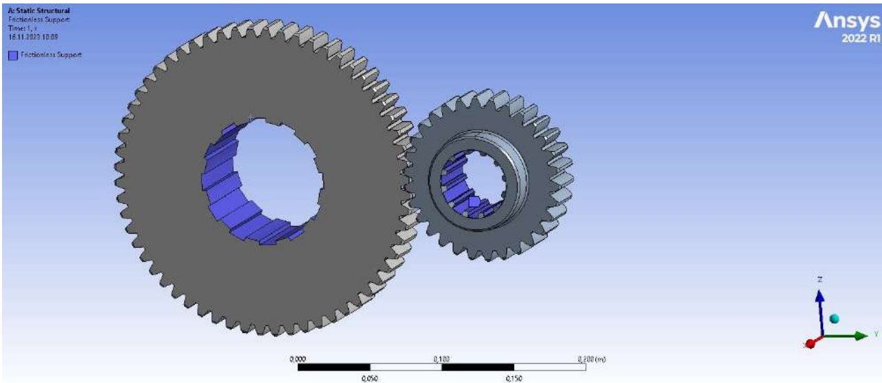
Рис. 3. Граничные условия на прямозубом приводе
