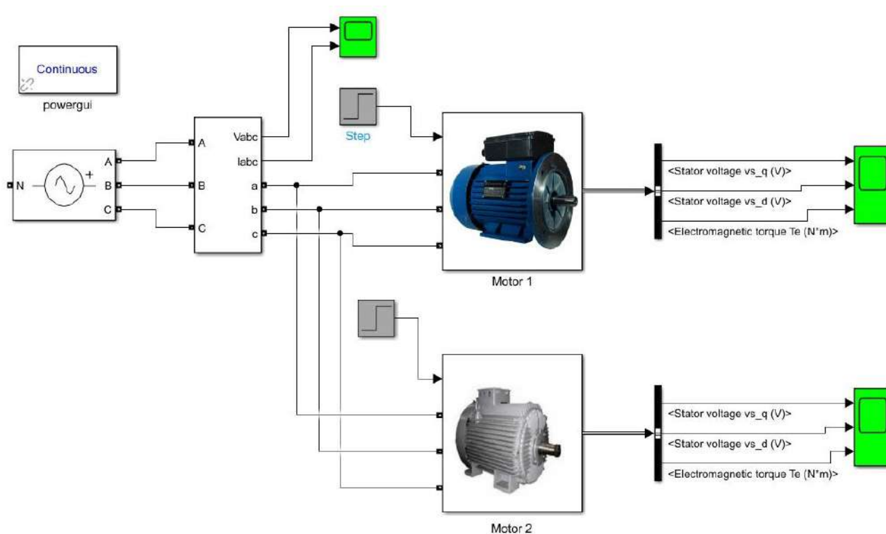
3-rasm. Elektr motorning Matlab/Simulink muhitda visual sxemasi
