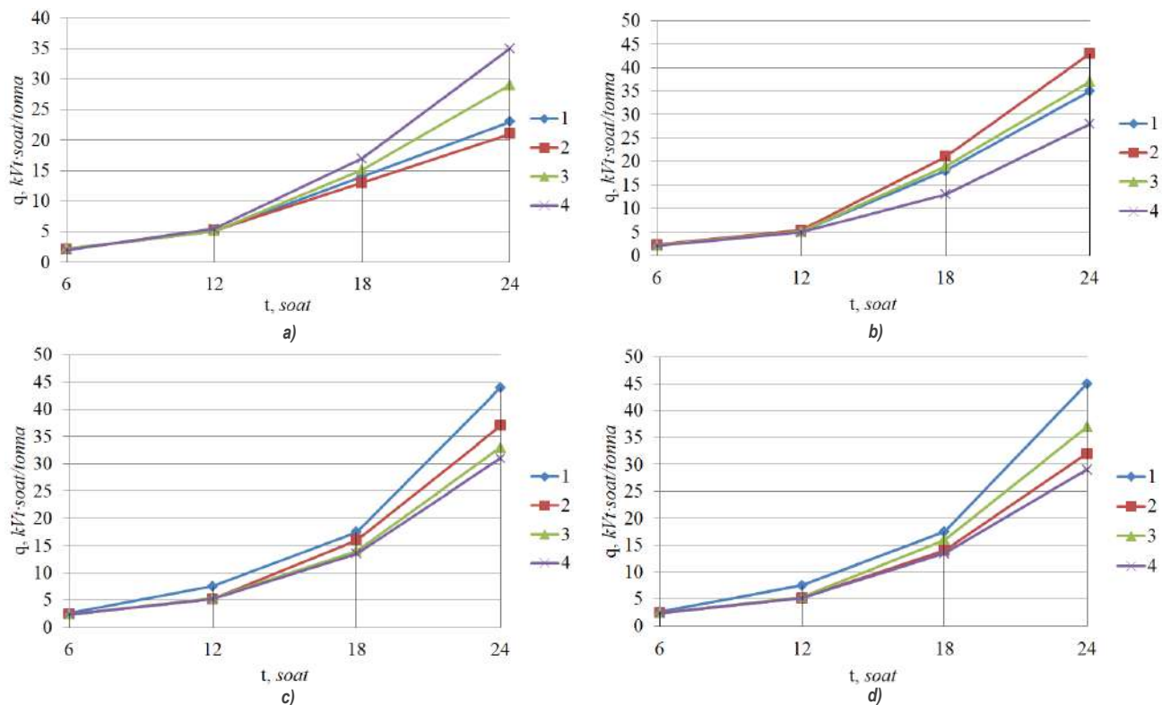
4-rasm. Solishtirma elektr energiya sarfini yanchish vaqtiga eksperimental bog'liqligi: a) 1-aylanish tezligi uchun; b) 2-aylanish tezligi uchun; c) 3-aylanish tezligi uchun; d) 4-aylanish tezligi uchun
