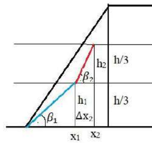
Рис. 3. Схема определения рационального угла откоса второго подступа
