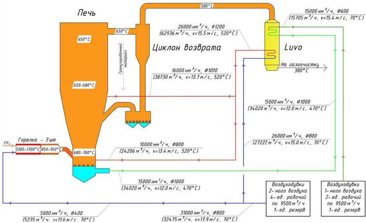
Рис. 2. Существующая схема работы печи кипящего слоя на ГМЗ-3
