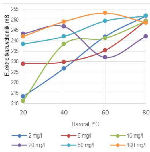
4-rasm. Elektr o'tkazuvchanligini PAA konsentratsiyasiga turli haroratlardagi bog'liqligi
