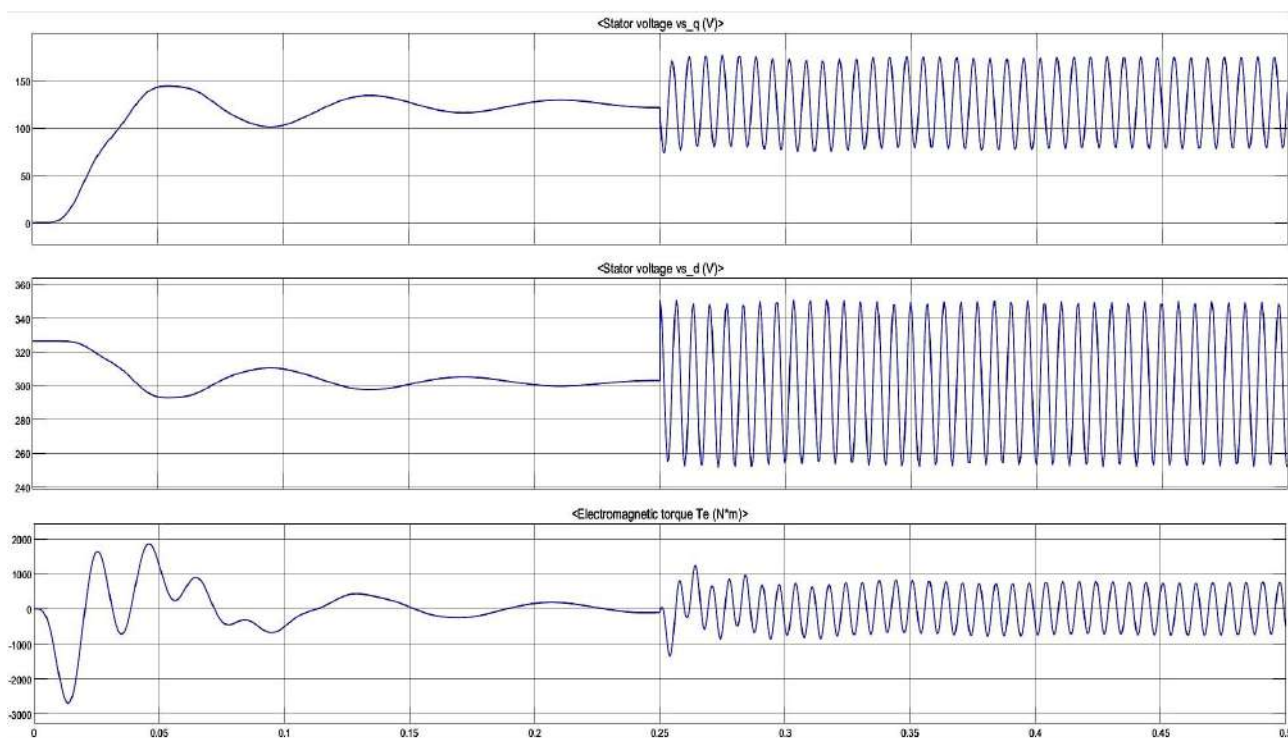
5-rasm. Ikkinchi elektr motorning d va q o'qlar bo'yicha kuchlanishlari hamda aylantiruvchi momentning o'zgarish grafigi (a, b, v)
