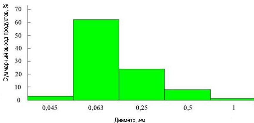
Рис. 2. Гранулометрический состав измельчённого технического углерода
