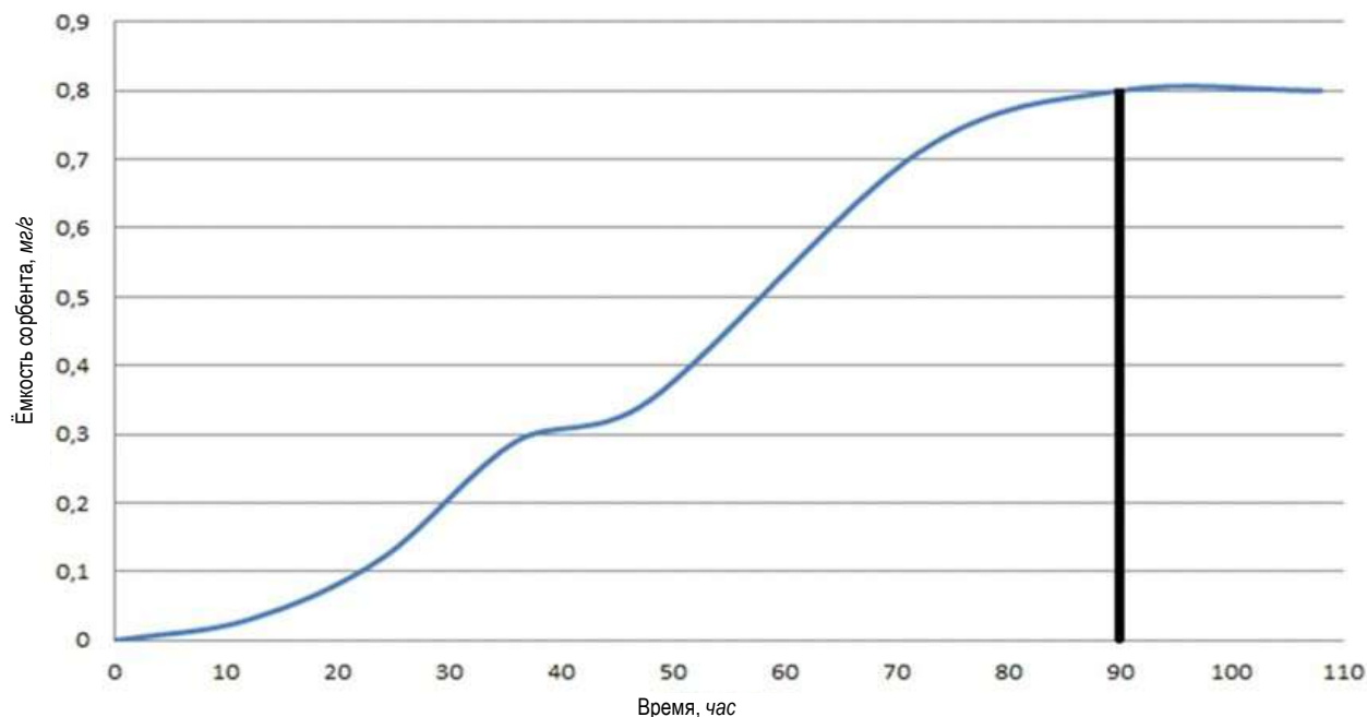
Рис. 2. Зависимость насыщения сорбента золотом от времени сорбции из оборотной воды с исходной концентрацией C_{исх.} = 0,035 мг/л
