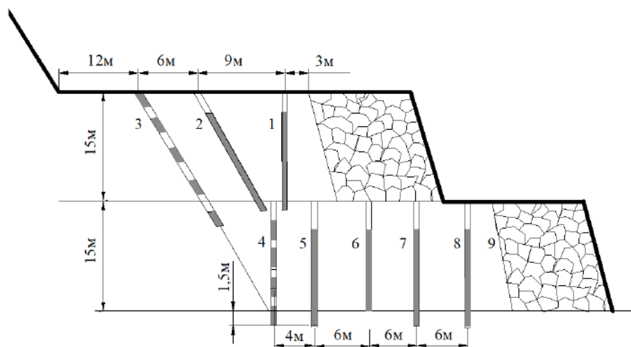
Рис. 5. Сдвигание уступов при падении трещин в сторону массива
