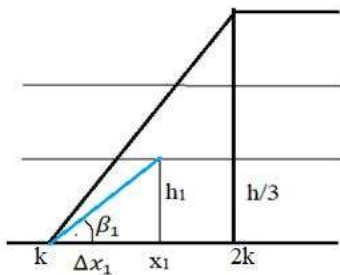
Рис. 2. Схема определения рационального угла откоса первого подступа
