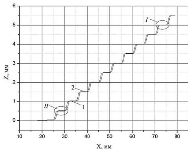
3-rasm. 1 va 2 ishlov berilgan yuzalarni o'lchangan holati
