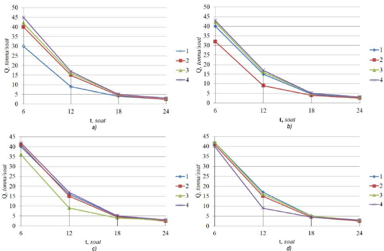
3-rasm. Unumdorlikni yanchish vaqtiga eksperimental bog'liqligi ko'rsatilgan: a) 1-aylanish tezligi uchun; b) 2-aylanish tezligi uchun; c) 3-aylanish tezligi uchun; d) 4-aylanish tezligi uchun
