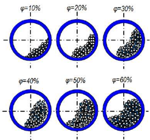
1-rasm. Markaziy bo'shatuvchi sharli tegirmonlarni shar bilan yuklanishlari (%)
