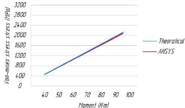
Рис. 8. Момент в зависимости от напряжения вон-Мизеса для Al
