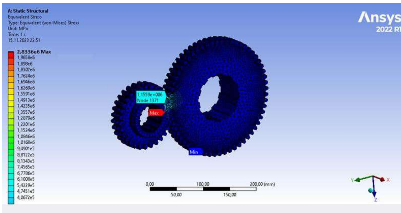
Рис. 5. Эквивалентное напряжение (вон-Мизеса)
