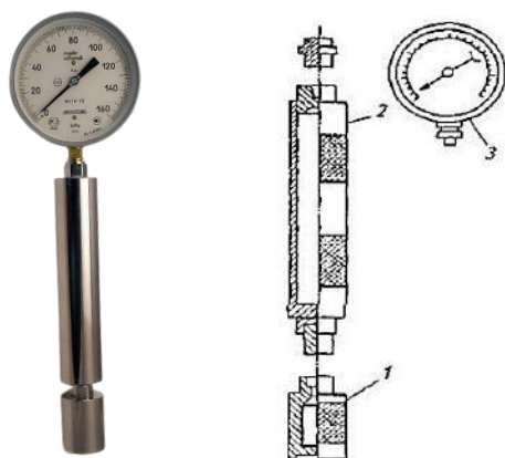
Рис. 1. Прибор Бомба-Рейда для определения давления насыщенных паров: 1 – топливная камера; 2 – воздушная камера; 3 – манометр
