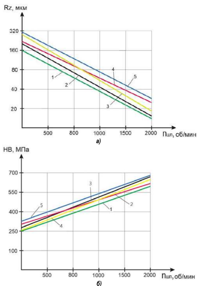
Рис. 4. Графики влияния режимов фрезерования с импульсным охлаждением на показатели качества обработанной поверхности: а – влияние частоты вращения шпинделя при различных значениях подачи на шероховатость; б – влияние частоты вращения шпинделя при различных значениях подачи на твердость; 1 – S_1 = 40 мм/мин; 2 – S_2 = 80 мм/мин; 3 – S_3 = 160 мм/мин; 4 – S_4 = 315 мм/мин; 5 – S_5 = 630 мм/мин
