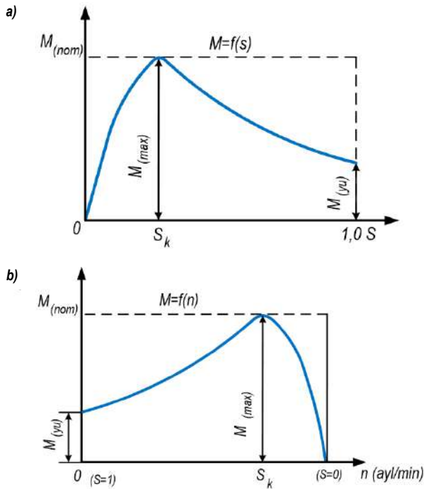
1-rasm. Sirpanish kamayganda elektr motorning aylantiruvchi momenti: a - elektr motorning sirpanish bo'yicha qurilgan mexanik xarakteristikasi; b - elektr motorning rotor aylanish tezligi bo'yicha qurilgan mexanik xarakteristikasi
