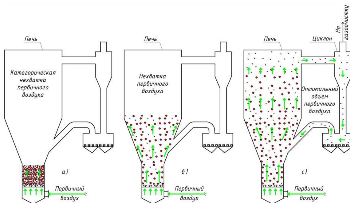
Рис. 1. Принципиальная схема формирования работы печи кипящего слоя: а – при категорической нехватке первичного воздуха; в – при нехватке первичного воздуха; с – при подаче оптимального объема первичного воздуха
