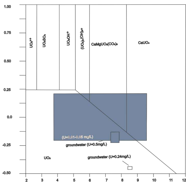
Рис. 3. Eh-pH диаграмма урана (0,01-0,5мг/л) в доломитовой воде
