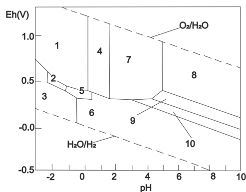
Рис. 5. Диаграмма Eh-pH и формы нахождения урана в присутствии сульфатов: при t=25^\circ C , концентрация ионов-урана 0,01 мг/л; концентрации сульфат-ионов: 0,1 мг/л (1) UO_2^{2+} ; (2) U(SO_4)_2^{2-} ; (3) U^{4+} ; (4) UO_2(SO_4) ; (5) UO_2 ; (6) UO_2(SO)_2^{2-} ; (7) UO_2(OH)_2 \cdot H_2O ; (8) U_3O_8 ; (9) U_3O_9 ; (10) U_4O_9
