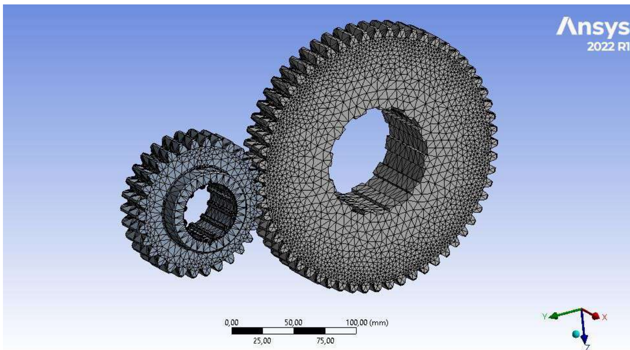
Рис. 2. Типичный вид прямозубой шестерни с зацеплением
