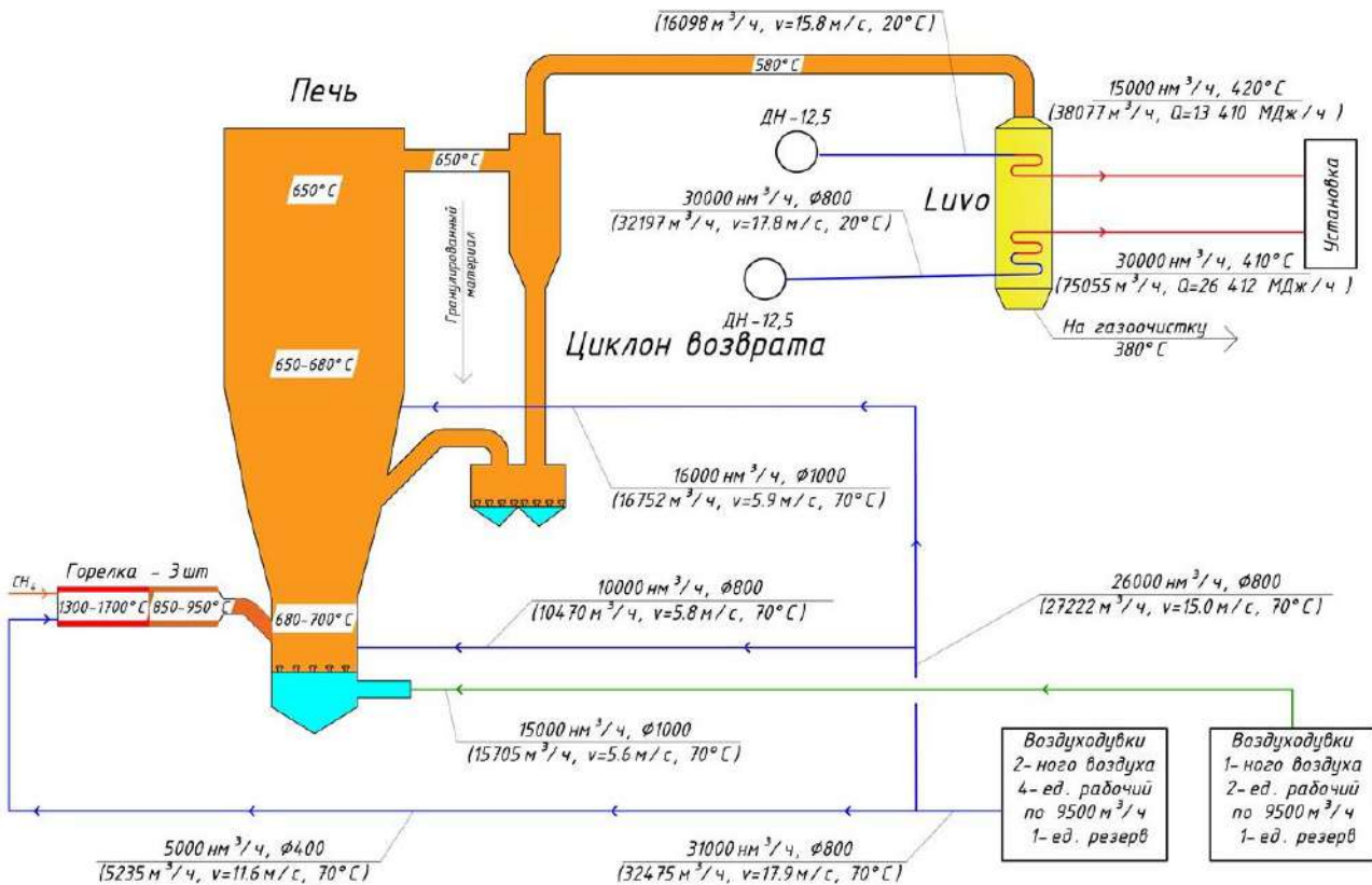
Рис. 3. Планируемая схема работы печи кипящего слоя на ГМЗ-3
