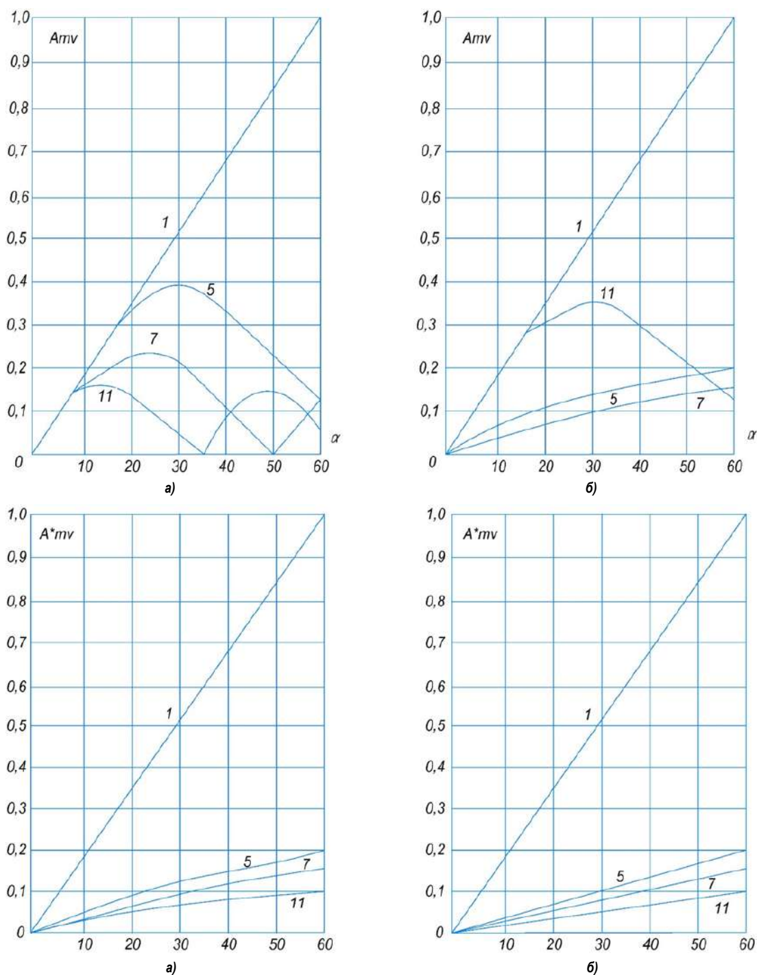
Рис. 3. Кривые характеризующие относительный гармонический состав линейного напряжения АИН с ШИР1: \eta=1 (а), \eta=2 (б), \eta=3 (в), \eta=4 (г)
