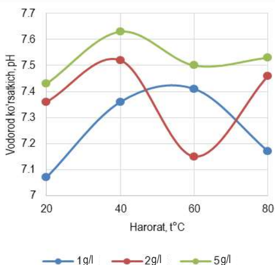
1-rasm. Bentonit suvli suspenziyasini (1 g, 2 g, 5 g) turli haroratlardagi pH qiymatini o'zgarishi
