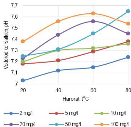
3-rasm. pH ni PAA konsentratsiyasiga turli haroratda bog'liqligi
