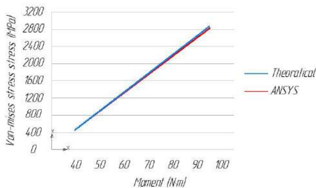
Рис. 6. Момент в зависимости от напряжения вон-Мизеса для сталь 40X ГОСТ 4543-2016
