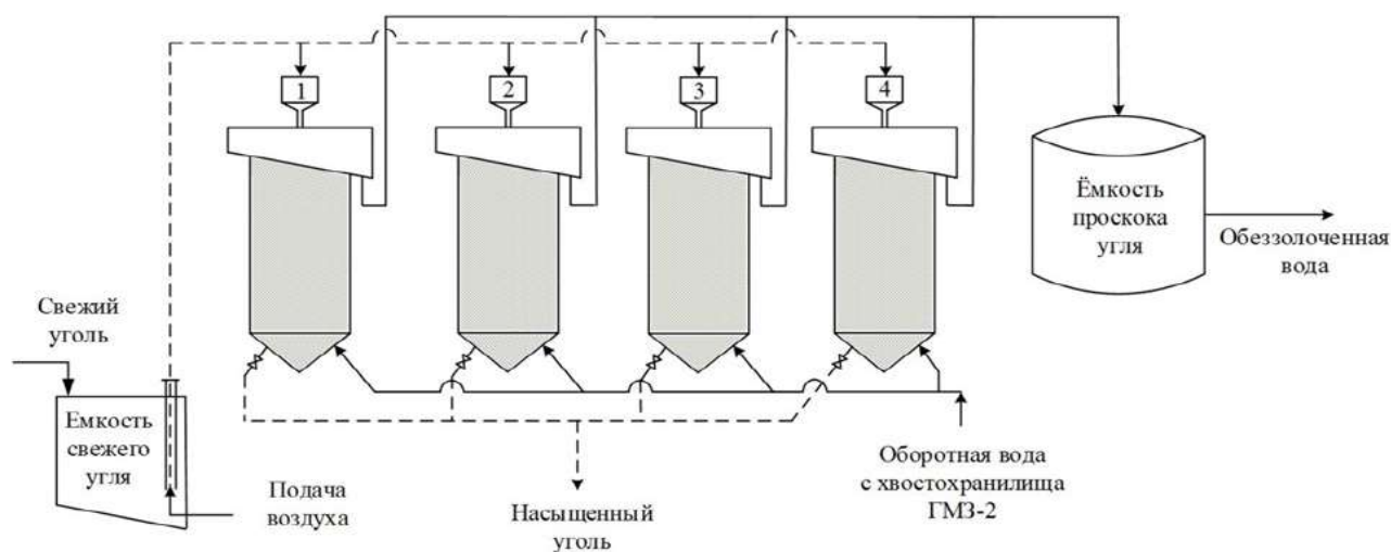
Рис. 3. Аппаратурная схема ЛСУ
