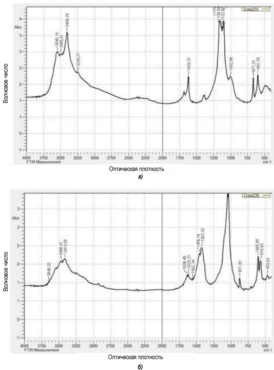
Рис. 2. ИК-спектры фосфогипса и фосфоритной руды месторождения Азнек: а) фосфогипс б) фосфорит
