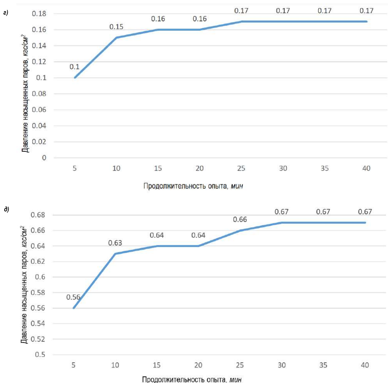
Рис. 1. Графики зависимости давления насыщенных паров нефти от продолжительности времени опыта на различных месторождениях: а – ЦПСН «Канибадам»; б – скважина № 22 Сельрохо (КИМ); в – скважина № 5 Махрам; г – скважина № 152 Нуязбек – Северный Каракчикум; д – бензин АИ – 92
