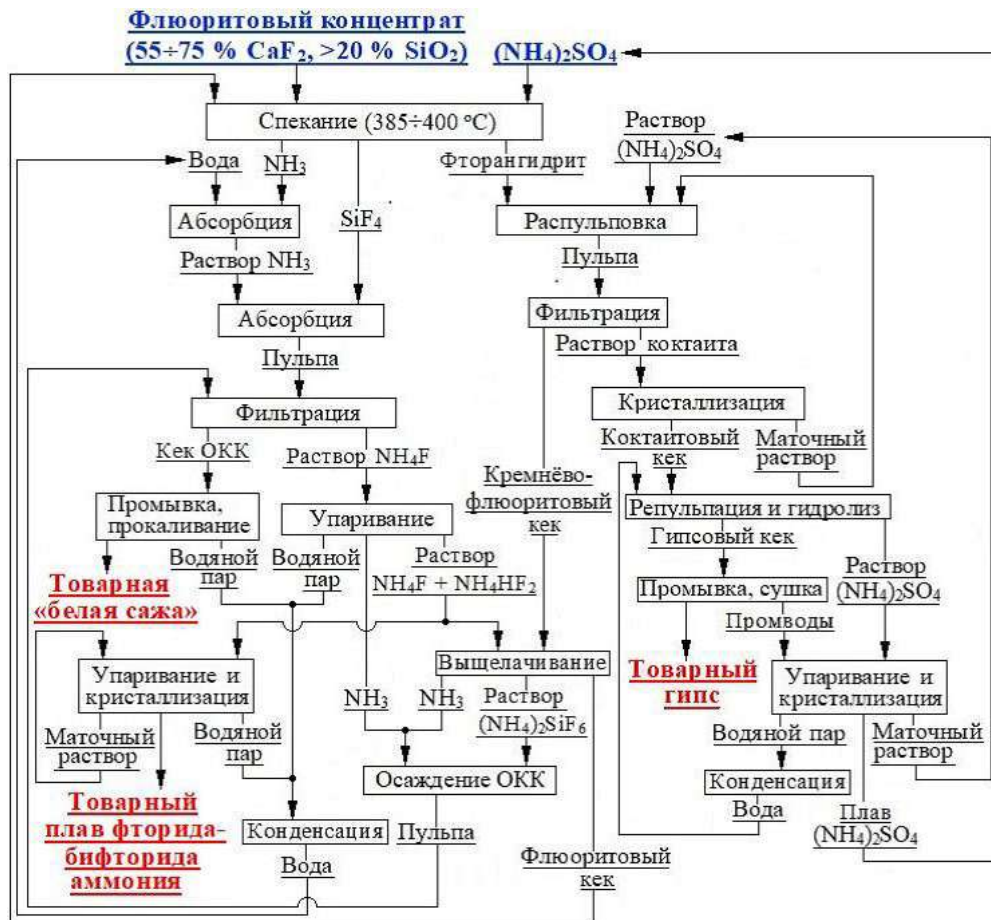
Рис. 2 Технологическая схема процесса переработки metspar на ФБА, «белую сажу» и товарный гипс
