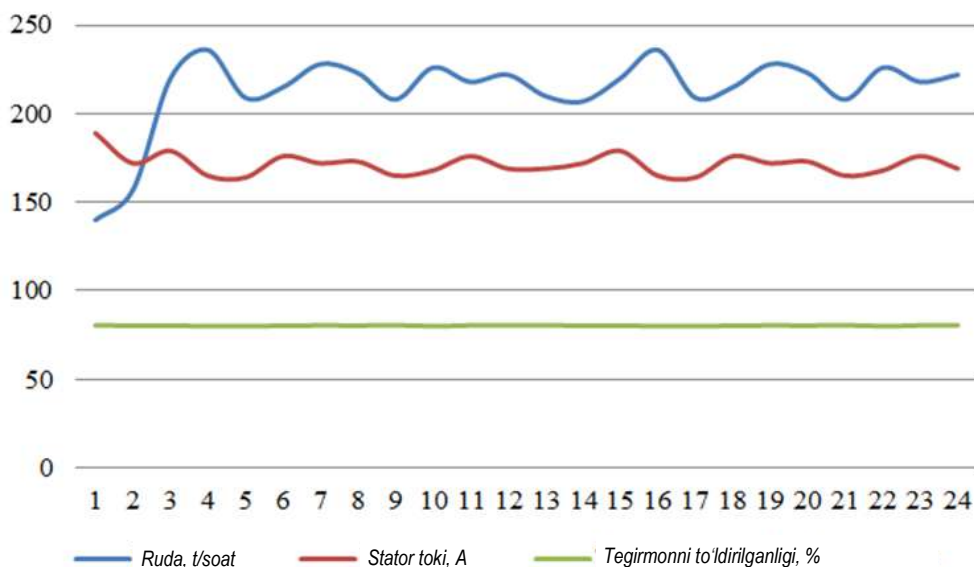
6-rasm. Markaziy bo'shatuvchi sharli tegirmonlarni nazorat qiluvchi shumamer qurilmasi ko'rsatkichlari
