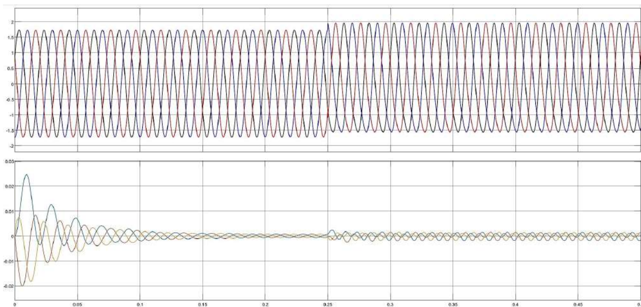
4-rasm. Ikkinchi elektr motorning iste'mol qiladigan tok va kuchlanishlarining o'zgarish grafigi
