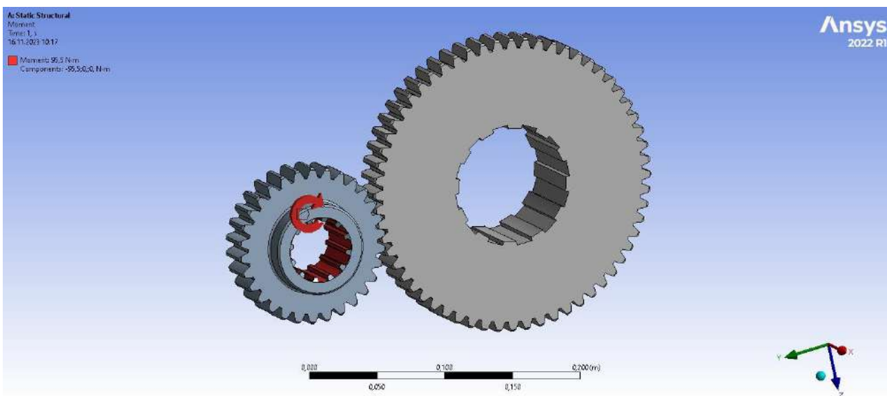
Рис. 4. Приложение момента к шестерне
