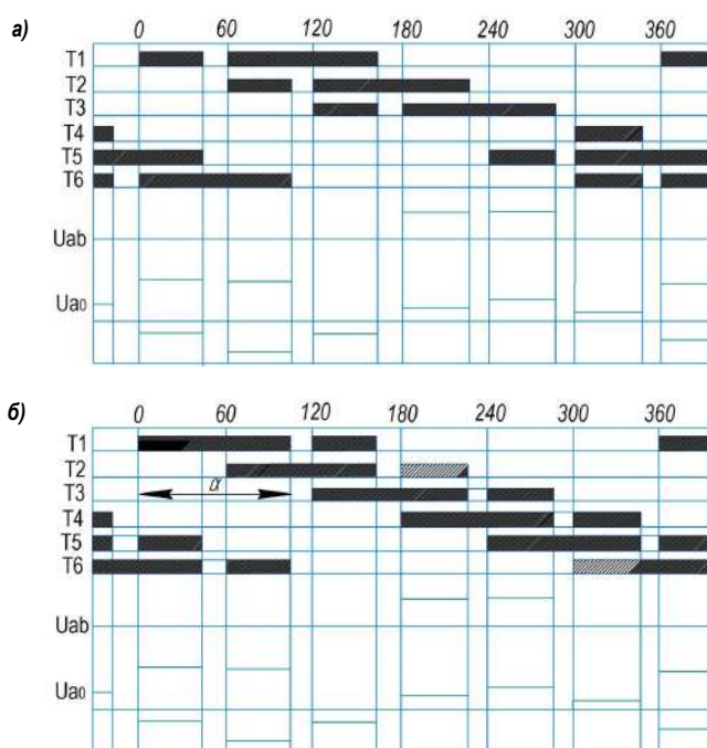
Рис. 1. Диаграммы состояний силовых тиристоров и кривые линейного и фазного напряжений
