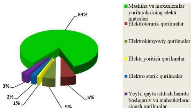
5-rasm. 2-sonli gidrometallurgiya zavodidagi energetik qurilmalar o'rtasida elektr energiyaning ulushlarda taqsimlanishi
