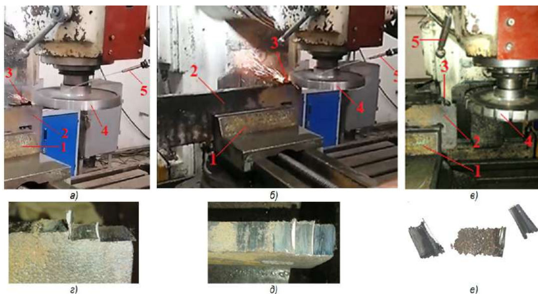
Рис. 3. Процессы термофрикционного фрезерования с импульсным охлаждением (некоторые обработанные образцы и стружки): а, б – процессы термофрикционного фрезерования с импульсным охлаждением; в – после остановки процесса обработки; г, д – некоторые обработанные образцы; е – стружки; 1 – тиски для зажима заготовки; 2 – заготовка из стали 110Г13Л; 3 – процесс образования стружки; 4 – фреза трения; 5 – трубка для подачи СОЖ
