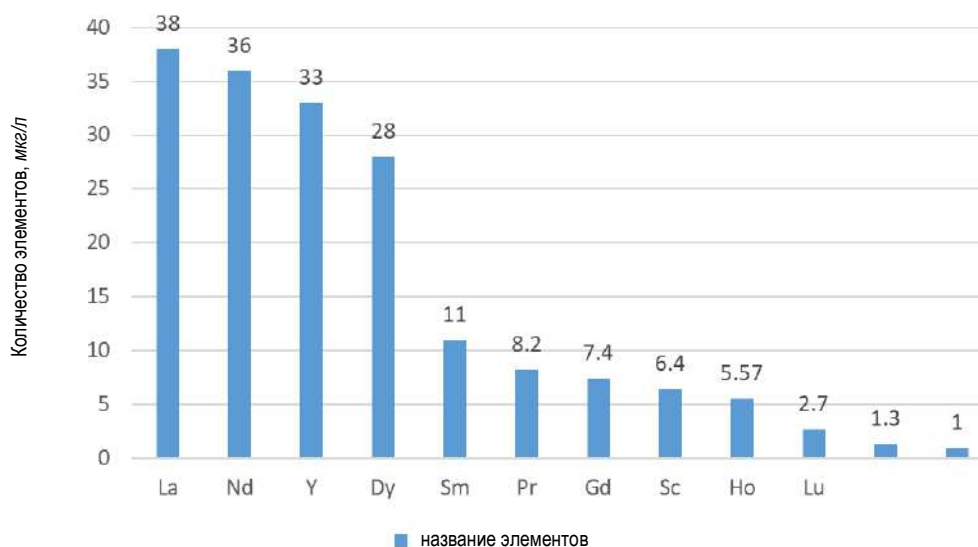
Рис. 1. Диаграмма снижения количество РЗЭ в составе экстракционной фосфорной кислоты
