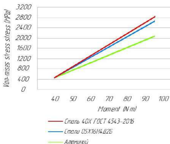
Рис. 9. Момент в зависимости от напряжения вон Мизеса для Сталь 40Х ГОСТ 4543-2016, нержавеющая Сталь 05Х16Н4Д2Б, и алюминий
