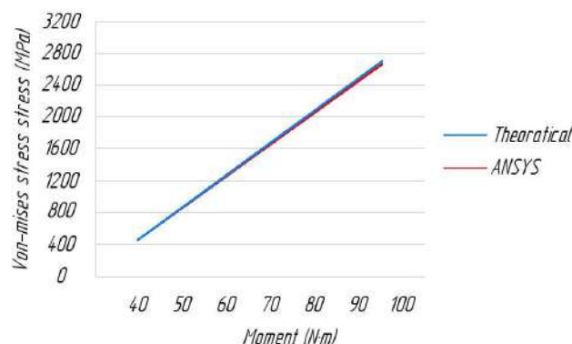
Рис. 7. Момент в зависимости от напряжения вон-Мизеса для Стали 05X16H4Д2Б
