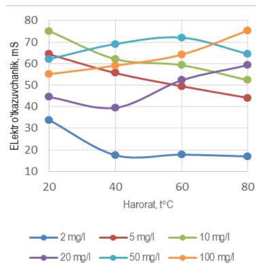
6-rasm. Elektr o'tkazuvchanligini kraxmal konsentratsiyasiga turli haroratlardagi bog'liqligi.
