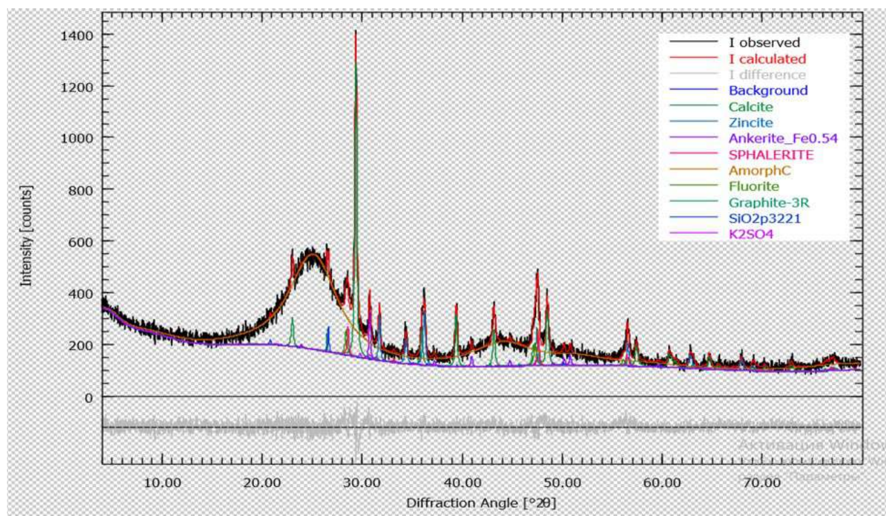
Рис. 3. Рентгенограмма углеродсодержащего материала, полученного пиролизом изношенных автомобильных шин
