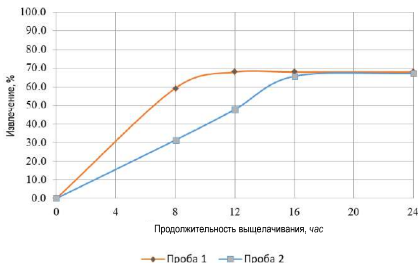
Рис. 1. Зависимость извлечения золота от продолжительности выщелачивания
