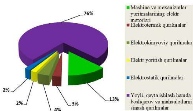
3-rasm. Navoiy mashinasozlik zavodidagi energetik qurilmalar o'rtasida elektr energiyaning ulushlarda taqsimlanishi
