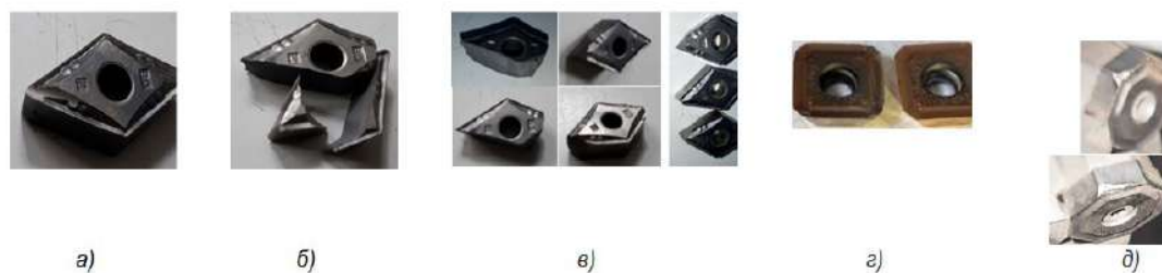
Рис. 1. Изношенные пластины различных производителей при обработке заготовки из стали 110Г13Л: а, б – пластины производства SANDVIK Coromant: новая пластина (а) и после первого прохода обработки (б), изношенные пластины (в); г – изношенные пластины производство компании Korloy (Южная Корея); д – сменные многогранные фрезерные пластины ONMU080612-YG613 Корейской компании YG-1
