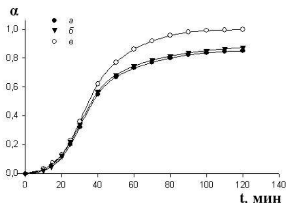
Рис. 1. Зависимость степени извлечения фтора \alpha от времени t (мин) при сернокислотном разложении флюорита при температуре 120°C (по данным [2]): а – минерал флюорит; б – флюоритовый концентрат ФК-92; в – минерал флюорит (или ФК-92) в присутствии \alpha -кварца
