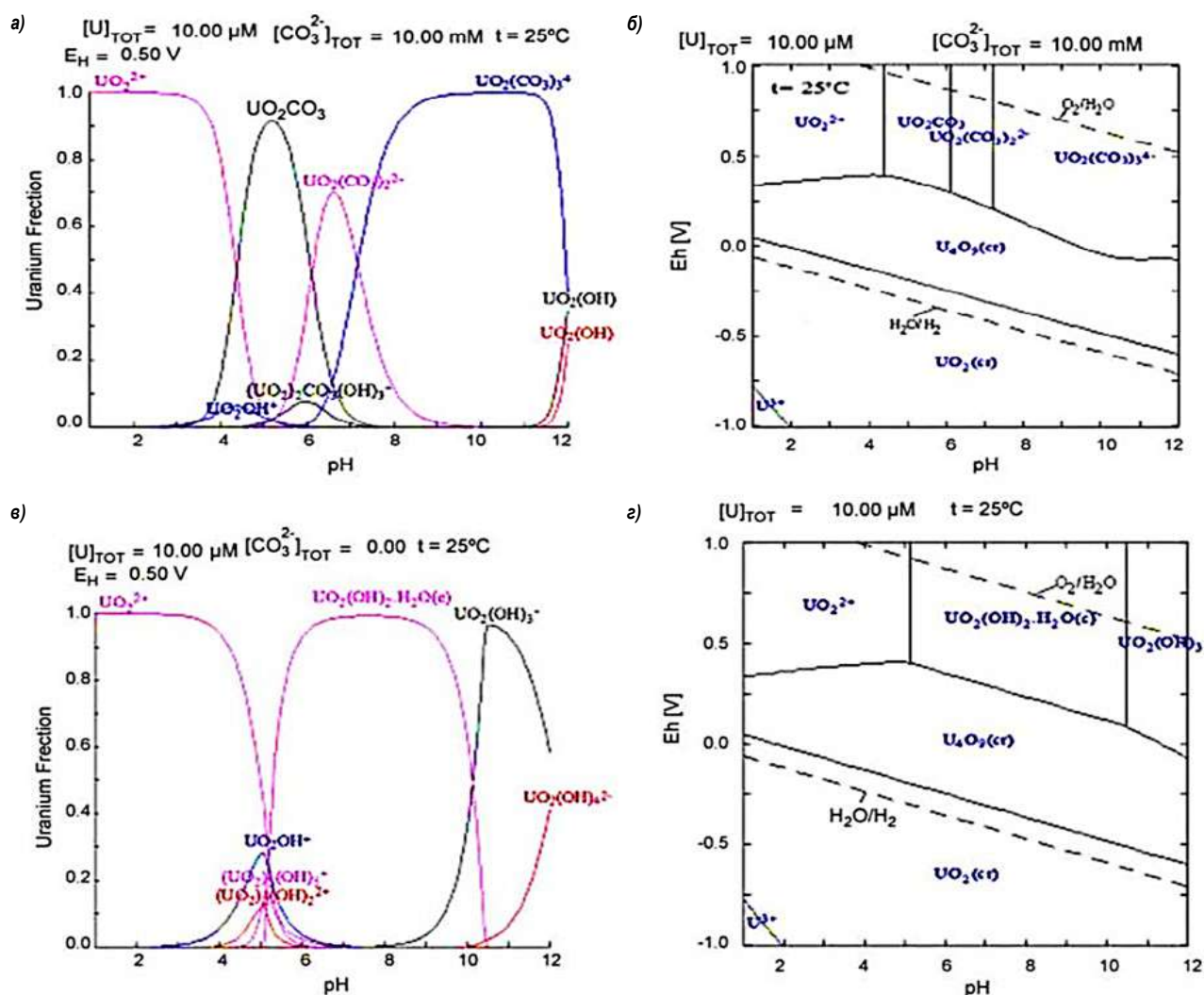
Рис. 1. Зависимость форм урана от Eh-pH (а-г)
