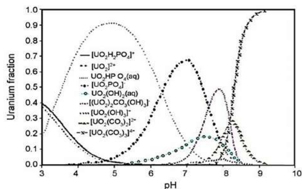
Рис. 4. Рассчитанные значения доли различных форм урана в системе UO_2-PO_4-CO_3-OH-H_2O при t=25^\circ C
