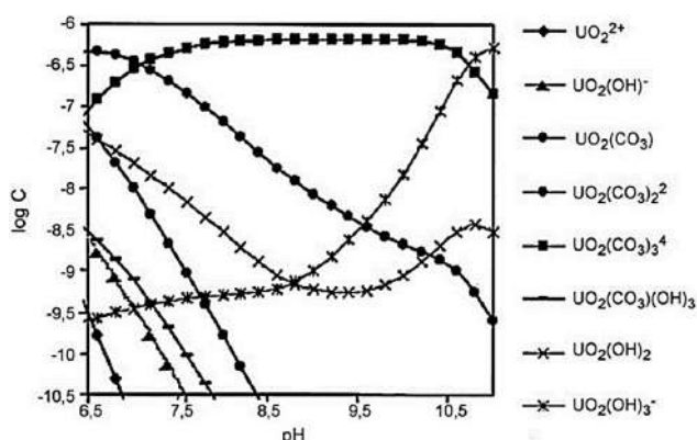
Рис. 2. Влияние pH и концентрации диоксида углерода на химические формы урана в природных водах
