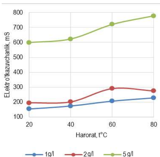
2-rasm. Bentonit suvli suspenziyalari (1 g, 2 g, 5 g) turli haroratlardagi elektr o'tkazuvchanligi
