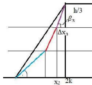
Рис. 4. Схема определения рационального угла откоса третьего подступа
