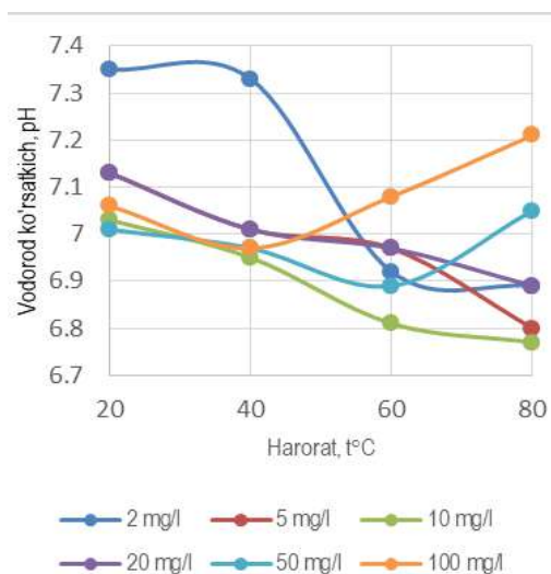
5-rasm. pH ni kraxmal konsentratsiyasiga turli haroratda bog'liqligi
