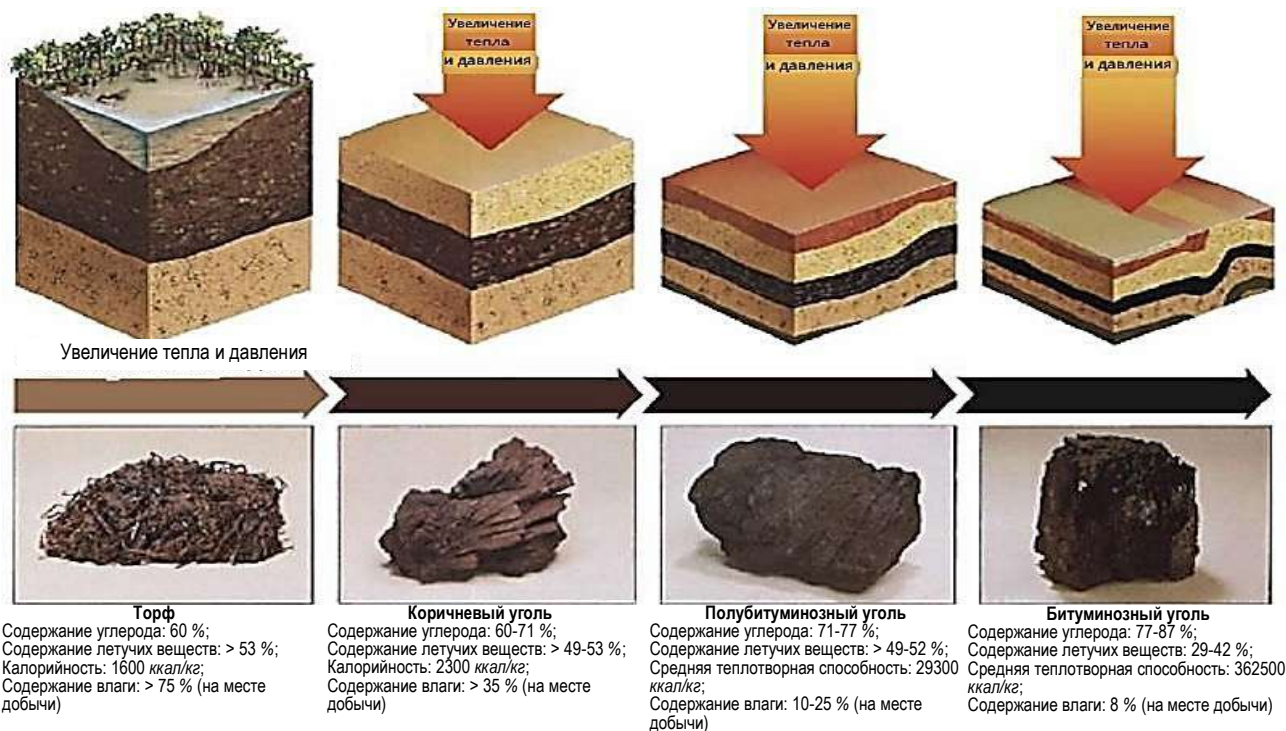
Рис. 1. Изменение свойств угля в зависимости от температуры и давления окружающей среды [4]
