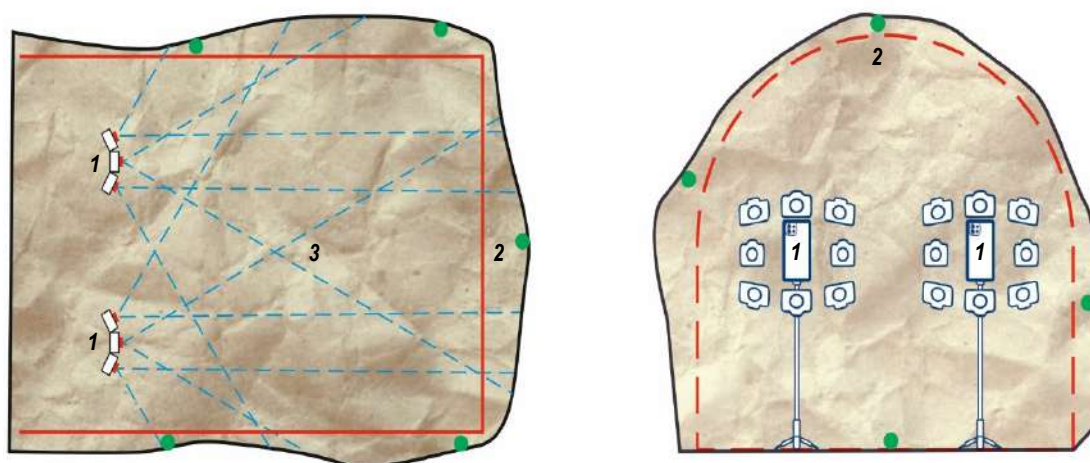
Рис 3. План-схема (слева) и разрез фотографирования (справа): 1 – мобильная камера; 2 – опорные точки; 3 – направление фотографирования
