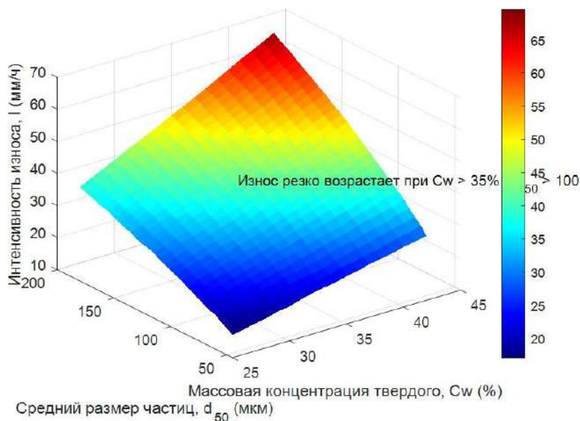
Рис. 1. Поверхность зависимости интенсивности износа от массовой концентрации твёрдого и среднего размера частиц
