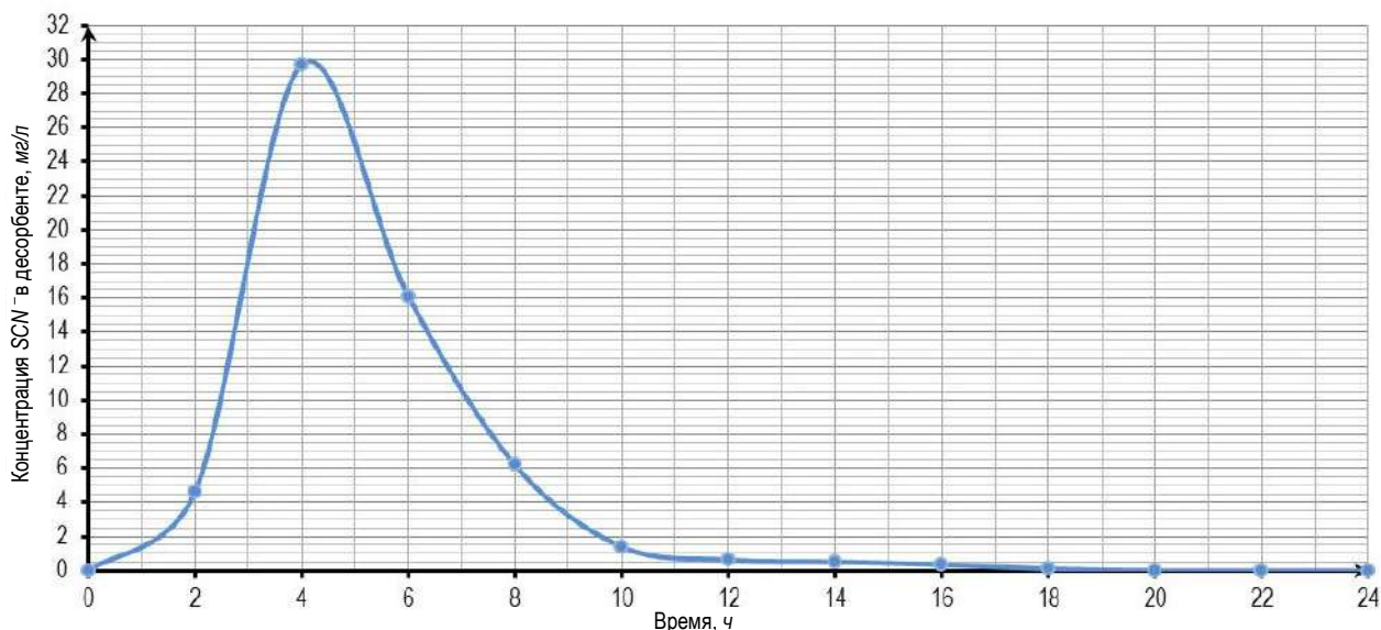
Рис. 3. График выходной кривой десорбции
