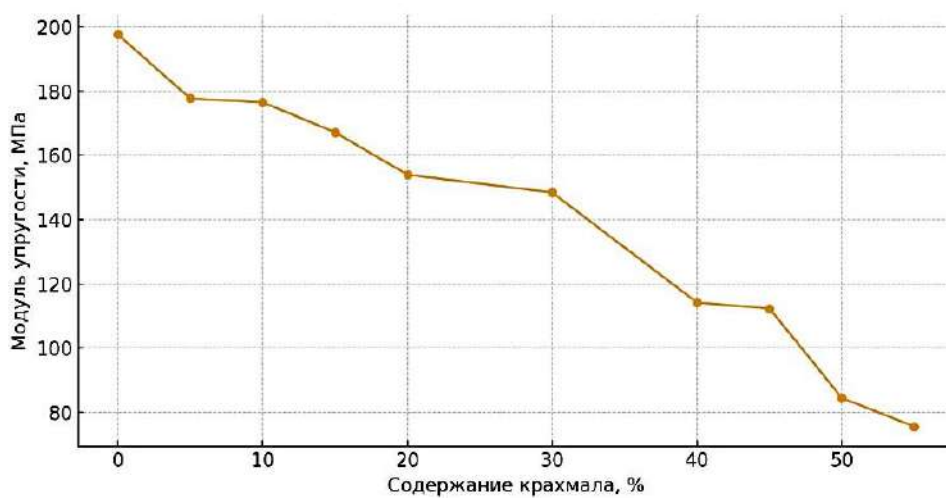
Рис. 3. Зависимость модуля упругости композитов ПЭНП/крахмал/МСГ от содержания модифицированного рисового крахмала
