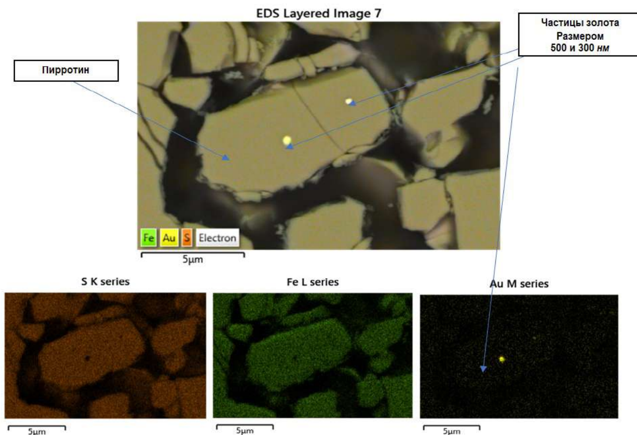
Рис. 2. ЭДС-карты распределения элементов, показывающие наночастицы золота (яркая точка на карте Au) в пирротине: карта распределения серы (S); карта распределения железа (Fe); карта распределения золота (Au)
