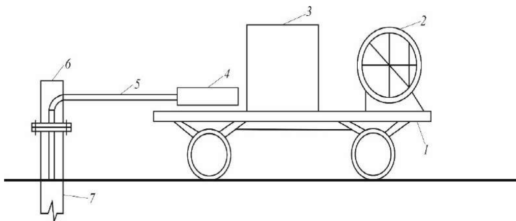
Рис. 2. Установка для подачи реагента: 1 – прицеп; 2 – барабан; 3 – ёмкость; 4 – химический насос; 5 – полиэтиленовая плетль; 6 – оголовок; 7 – технологическая скважина
