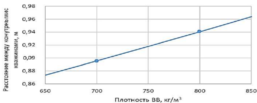
Рис. 14. Влияние плотности промышленных ВВ на изменение расстояния между контурными скважинами
