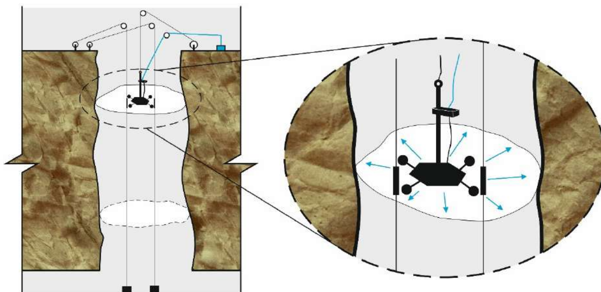
Рис. 1. Схема съёмки сечений (слева) и общий вид устройства проведения съёмки (справа): 1 – кабель к электрическому спусковому устройству затвора фотоаппарата (ДА-2); 2 – устройство для дистанционного управления кнопкой затвора; 3 – кабель к лампе-вспышке, кабель к длинномеру ДА-2, направляющая проволока; 6 – направляющая фото планиметр; 7 – свет от вспышки; 8 – световой след на стенке выработки
