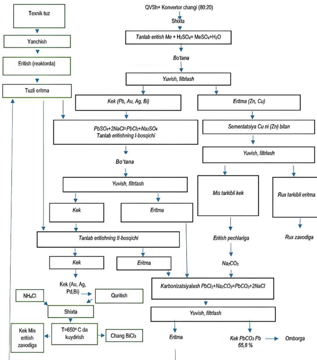
1-rasm. QVSh va mis eritish zavodi changini gidrometallurgik usulda qayta ishlash texnologik tasviri
