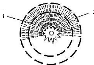
Рис. 1. Режим супердробления горных пород при взрыве заряда ВВ: 1 – передний фронт волны напряжений; 2 – задний фронт волны напряжений
