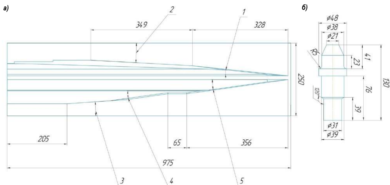
Рис. 2. Зубок РКС1.00.00.111 (а) горнопроходческого комбайна и клиновидный инструмент (б) для его прокатки на стане ПКП: 1 – упор, 2 – лоток, 3 – деформирующий клин, 4 – дорожки, 5 – деформирующий клин
