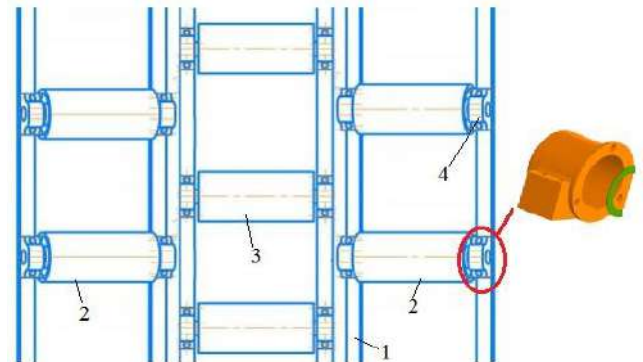
4-rasm. Rolik tayanchlariga rolidlarni o'rnatish va rolidlarga buksa qo'yish
