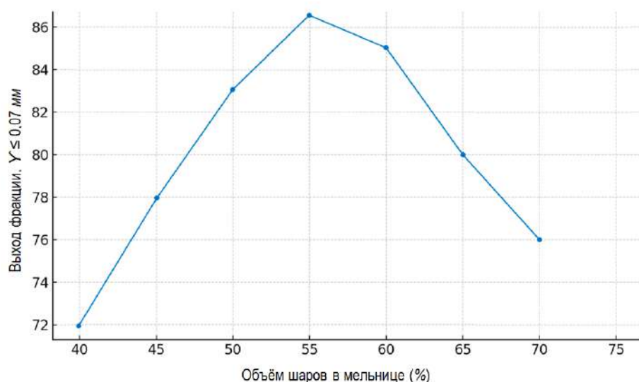
Рис. 4. Зависимость выхода готового продукта от объема загрузки шаров
