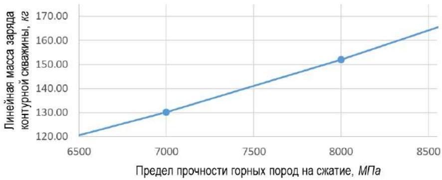
Рис. 10. Влияние предела прочности горных пород на сжатие на изменение линейной массы контурного заряда
