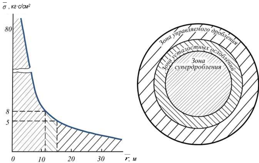
Рис. 4. Зоны различной интенсивности дробления в крепких горных породах при взрыве одиночного заряда
