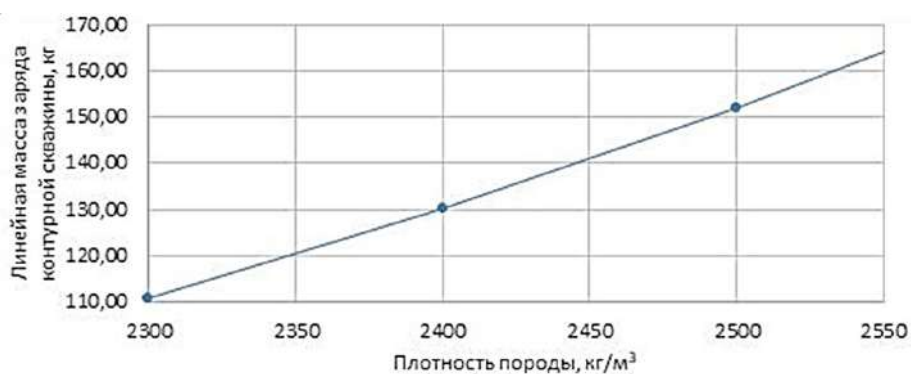
Рис. 6. Влияние плотности горных пород на изменение линейной массы заряда контурной скважины
