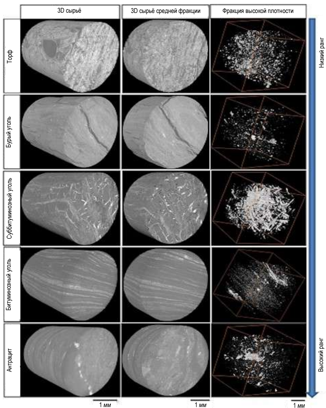
Рис. 3. 3D-визуализации микро-КТ изображений исследуемых углей
