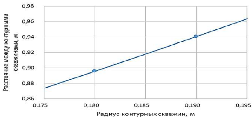
Рис. 16. Влияние радиуса контурных скважин на изменение расстояния между ними
