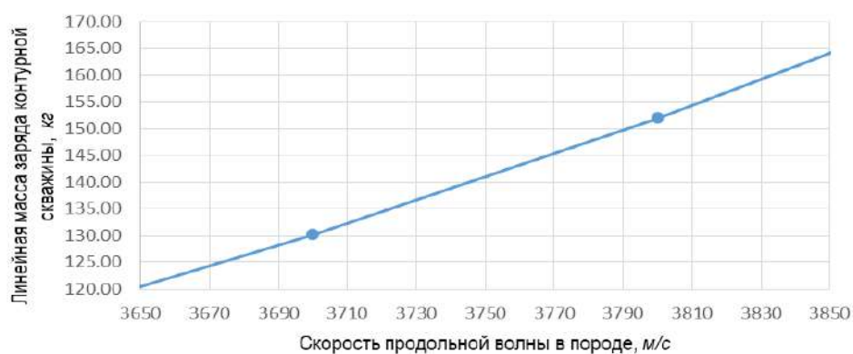
Рис. 7. Влияние скорости продольной волны в горной породе на изменение линейной массы контурного заряда
