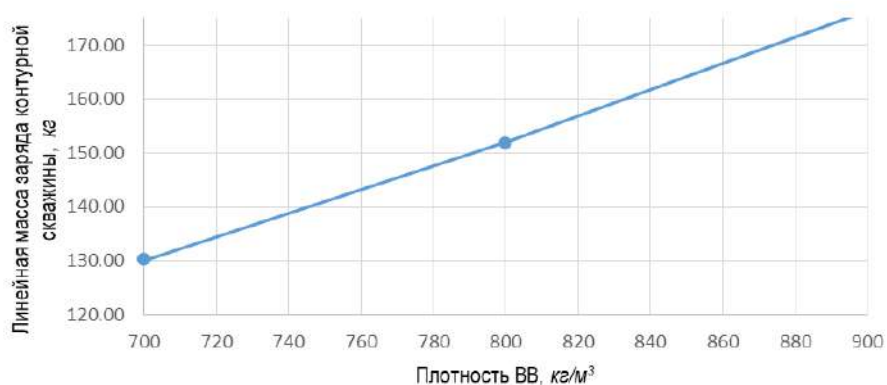
Рис. 8. Влияние плотности взрывчатого вещества на изменение линейной массы контурного заряда
