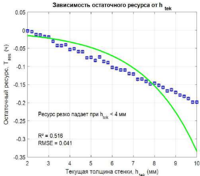
Рис. 4. Зависимость остаточного ресурса от текущей толщины стенок
