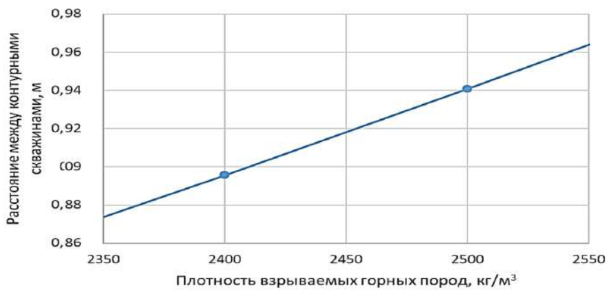
Рис. 12. Влияние плотности взрывааемых горных пород на изменение расстояния между контурными скважинами
