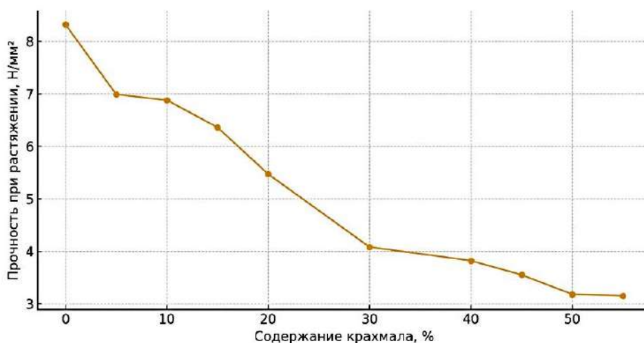
Рис. 1. Зависимость прочности при растяжении композитов ПЭНП/крахмал/МСГ от содержания модифицированного рисового крахмала
