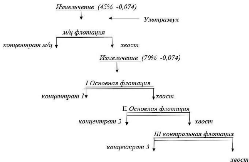
Рис. 1. Схема флотации с УЗО перед межцикловой флотацией
