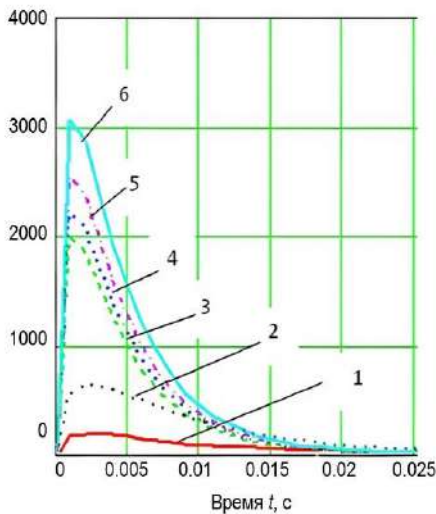
Рис. 2. Изменение скоростей смещения при разрушении породы скважинным зарядом с пеногелевой забойкой: а – общий вид; б – по логарифмической шкале; 1 – в породе; 2 – в забойке из буровой мелочи; 3, 4, 5, 6 – в пеногелевой забойке в зависимости от её плотности
