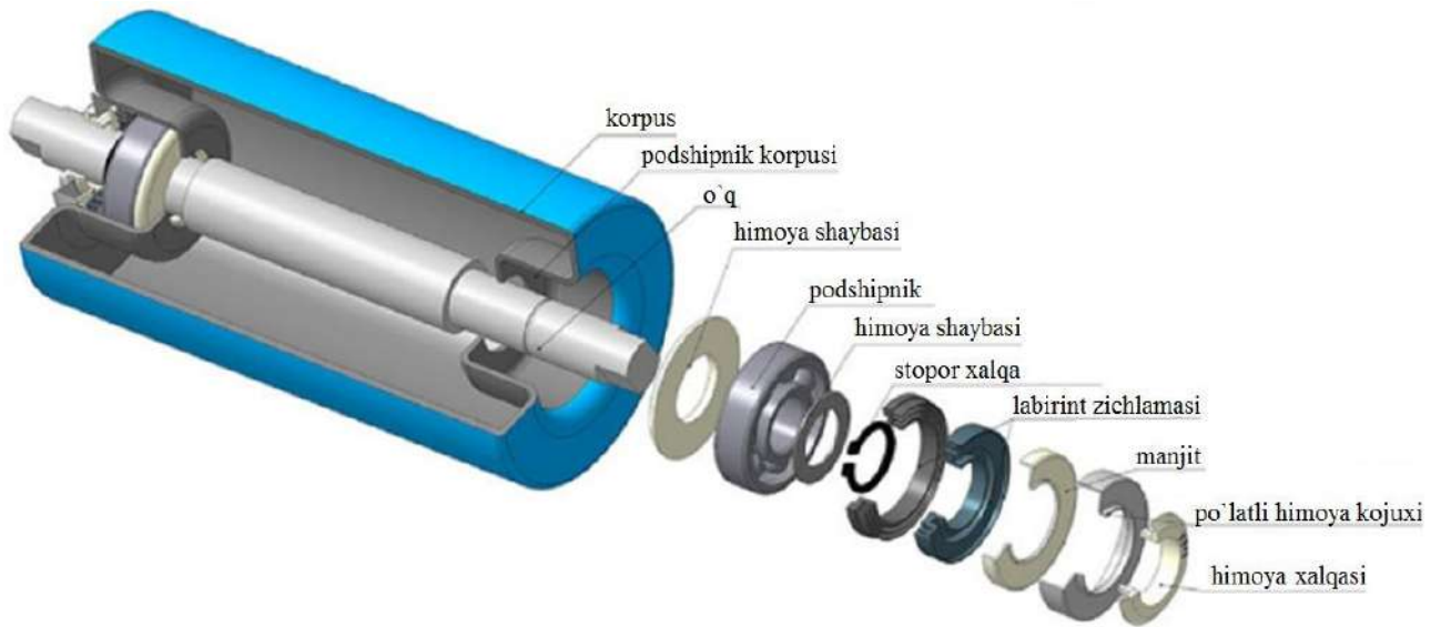
2-rasm. Rolikning asosiy qismi
