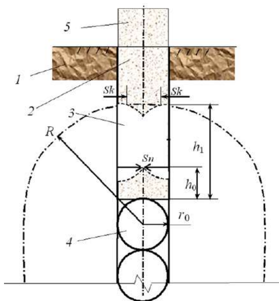
Рис. 3. Схема запирания канала скважины разрушенной породой при взрыве скважинного заряда: 1 – зона интенсивной трещиноватости; 2 – пеногелевая забойка переменного агрегатного состояния; 3 – зона запирания канала; 4 – заряд ВВ; 5 – пеногель, выдавленный из устья скважины; r_0 – радиус заряда; R – радиус зоны трещинообразования; h_0 – высота сжатия пеногелевой забойки; h_1 – расстояние до границы запирания; S_n – смещения частиц породы при выравнивании скоростей; S_k – смещения частиц породы при критической скорости
