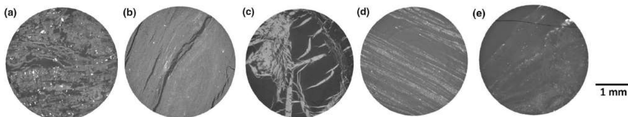
Рис. 2. 2D-изображения поперечного сечения микро-КТ различных образцов угля [5]: а) торф; б) лигнит; в) суббитуминозный; д) битумный; е) антрацит
