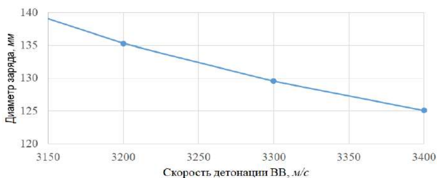
Рис. 5. Влияние скорости детонации ВВ на изменение диаметра контурного заряда
