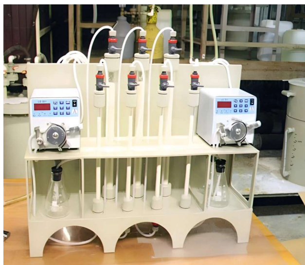
Рис. 1. Лабораторная установка для проведения исследований сорбционных процессов в динамических условиях
