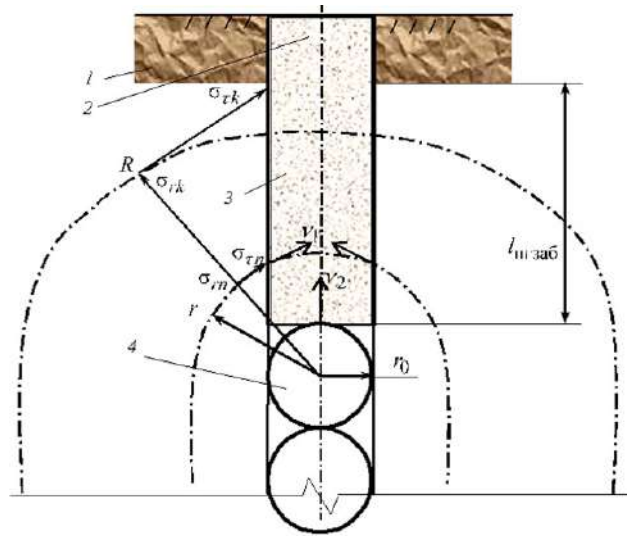
Рис. 1. Схема развития процесса смещения породы и пеногелевой забойки при взрыве скважинного заряда: 1 – зона интенсивной трещиноватости; 2 – пеногелевая забойка переменного агрегатного состояния; 3 – зона смещения породы из стенки скважины; 4 – заряд ВВ; r_0 – радиус заряда; r – радиус зоны смятия; R – радиус зоны трещинообразования; \sigma_r, \sigma_{rk}, \sigma_{\theta}, \sigma_{\theta k} – радиальные и тангенциальные составляющие волны сжатия в начале и на границе зоны трещинообразования; l_{заб} – длина пеногелевой забойки; v_1 – направление скорости смещения стенки скважины; v_2 – направление скорости смещения пеногелевой забойки
