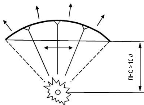
Рис. 2. Квазистационарный режим разрушения горных пород при взрыве заряда ВВ
