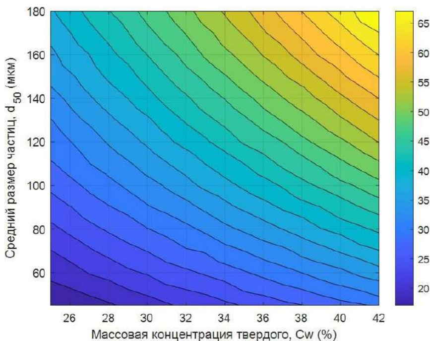
Рис. 2. Контурная диаграмма интенсивности износа от C_w и d_{50}
