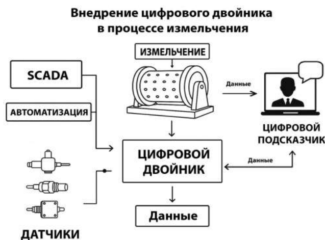
Рис. 1. Схема архитектуры системы цифрового двойника и цифрового подсказчика
