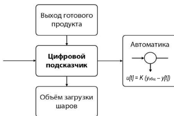
Рис. 3. Блок-схема алгоритма работы цифрового подсказчика
