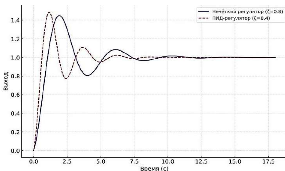
Рис. 4. Сравнение нечёткого логического контроллера и ПИД-регулятора по характеристикам переходного процесса
