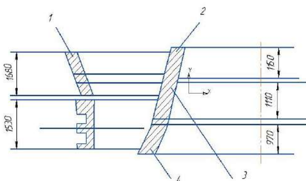
3-rasm. YKM-1500/300 yirik konusli maydalagichning zirhlari ni joylashtirish sxemasi: 1 – konusni zirhlari; 2, 3, 4 – yuqori, o'rta va pastki konusning zirhlari
