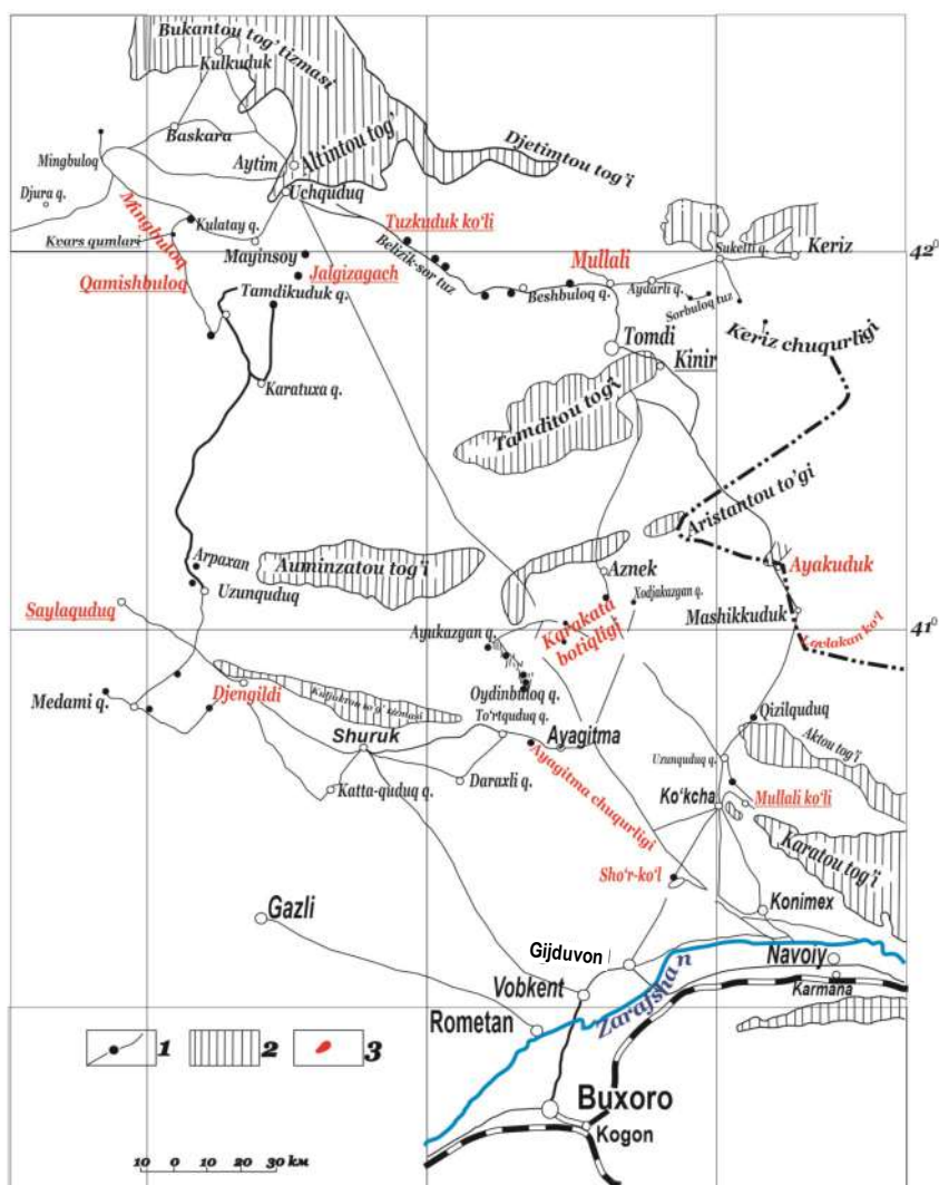
1-rasm. Markaziy Qizilqumda zamonaviy tuz qatlamlarining tarqalishiga doir sharhli xaritasi: 1 – shoʻrtanish hududlaridagi marshrutlar va kuzatuv nuqtalari; 2 – paleozoy davri togʻ jinslarining yuzaga chiqishi; 3 – eng yirik shoʻr koʻllar va konlar (chizib koʻrsatilgan)
