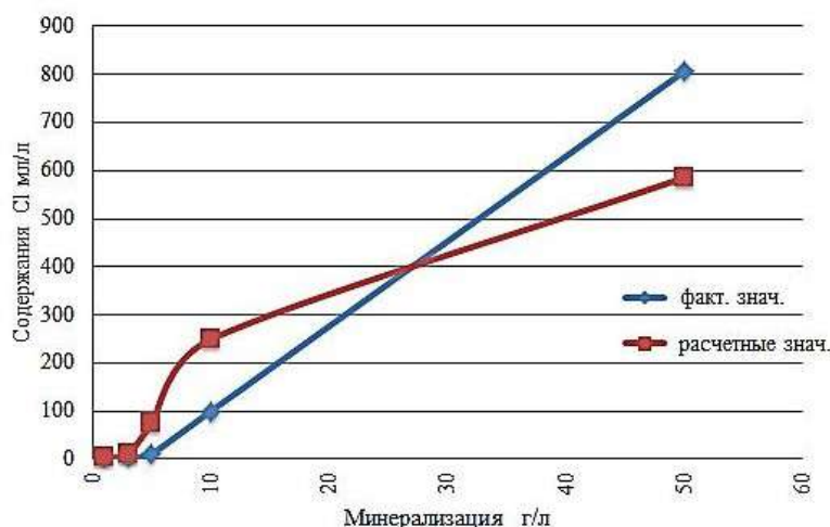
Рис. 3. Зависимость содержания Cl^- в поверхностных водах от минерализации в водах верхней гидродинамической зоны
