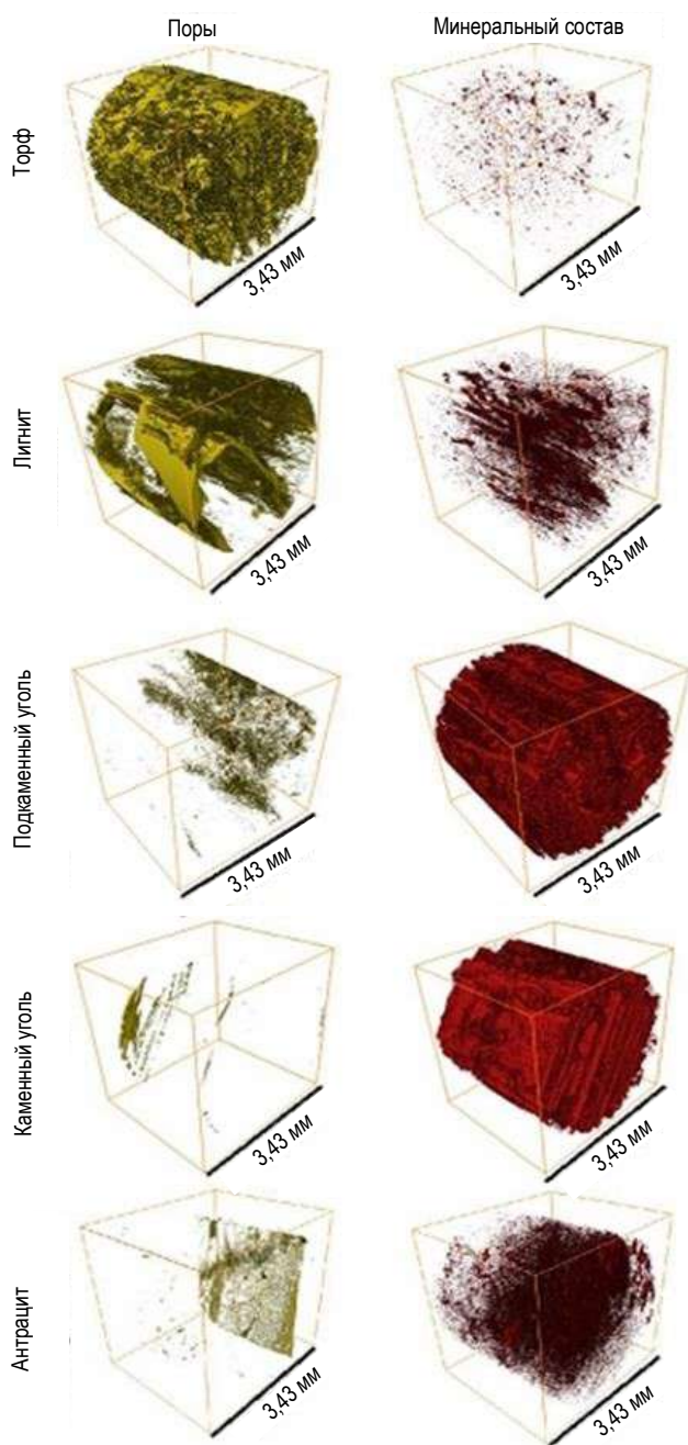
Рис. 5. 3D-морфология порового пространства и минерального вещества для каждой марки угля (номинальное разрешение 3,43 мкм)
