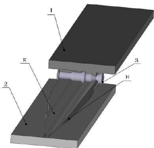
Рис. 1. Технологический процесс прокатки основы инструмента зубков горнодобывающих комбайнов с помощью программы QFORM: 1 – верхний клиновый инструмент; 2 – нижний клиновый инструмент; 3 – заготовка; Н – боковые наклонные грани; К – калибрующий участок
