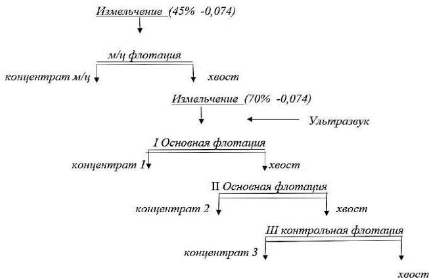
Рис. 2. Схема флотации с УЗО перед основной флотацией
