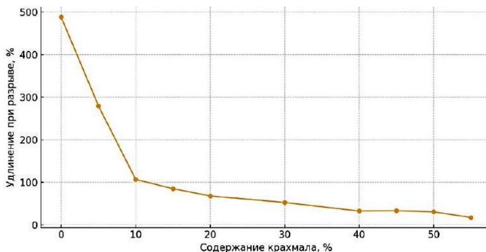
Рис. 2. Зависимость удлинения при разрыве композитов ПЭНП/крахмал/МСГ от содержания модифицированного рисового крахмала
