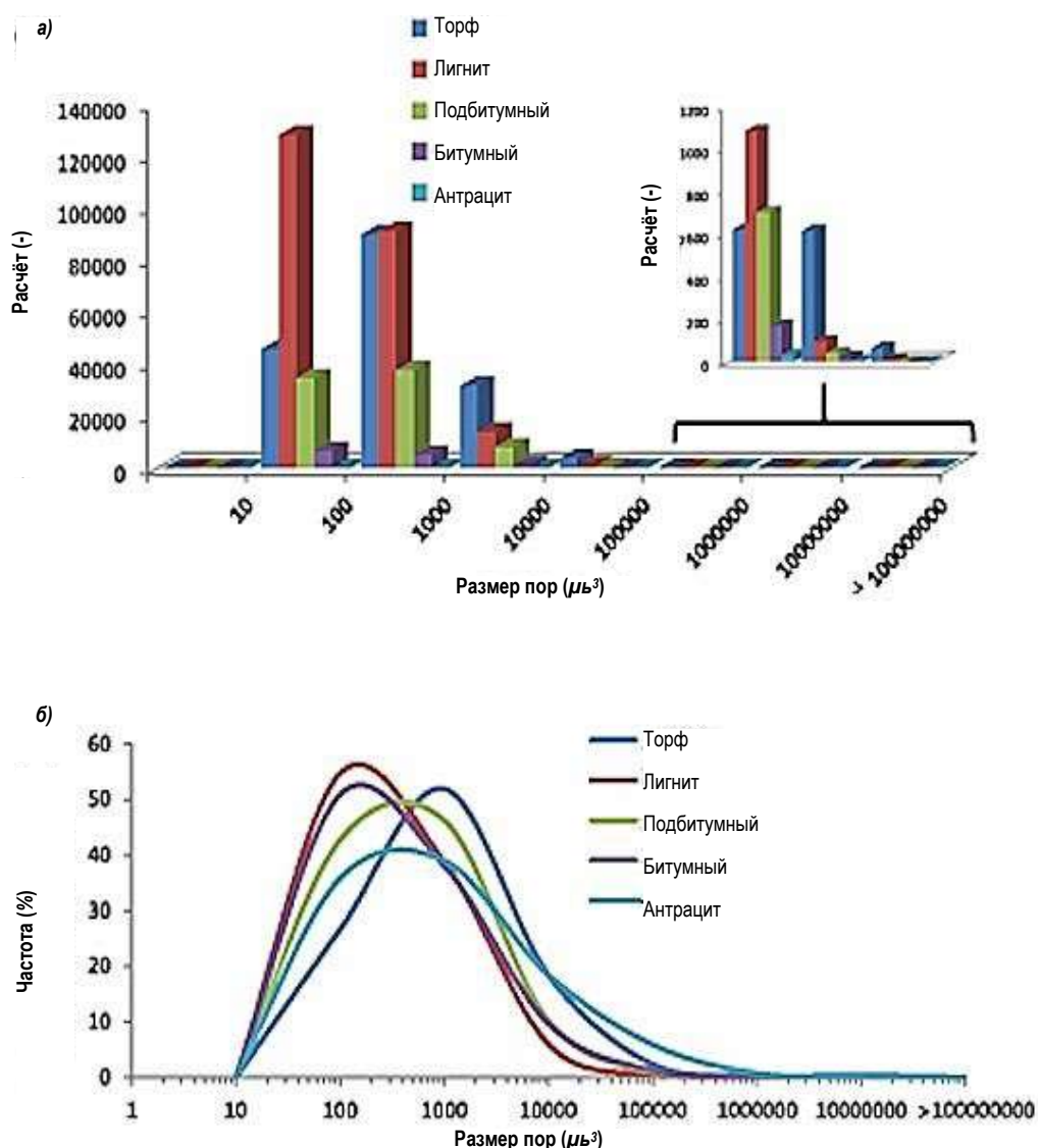
Рис. 6. Распределение размеров пор для образцов угля разной марки [5]: а – по количеству (-); б) – по частоте (%)
