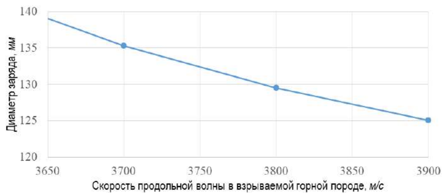
Рис. 4. Влияние скорости продольной волны в горной породе на диаметр контурного заряда
