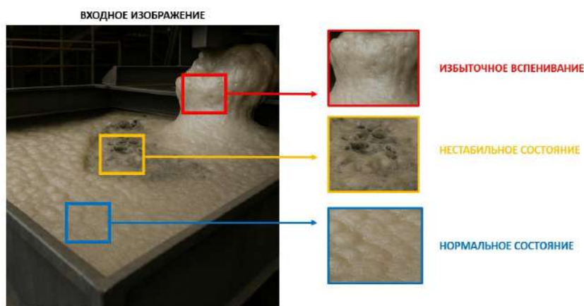
Рис. 2. Схема контроля состояния пены с применением свёрточных нейронных сетей
