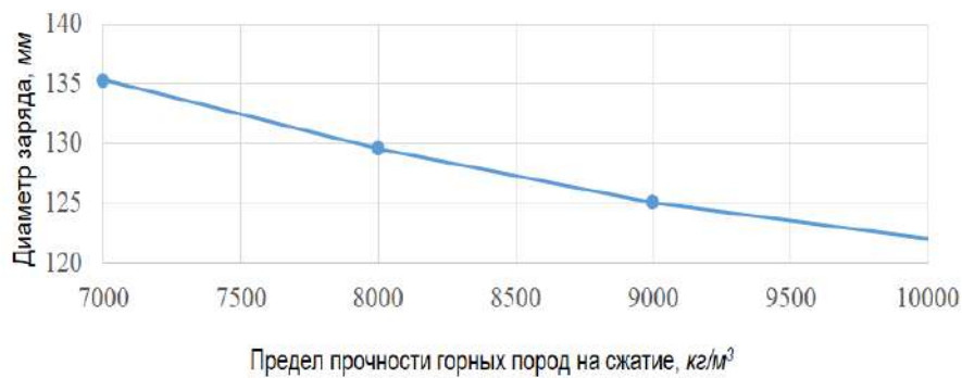
Рис. 3. Влияние предела прочности горных пород на сжатие на диаметр контурного заряда
