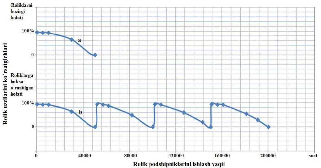
5-rasm. Rolik podshipniklarini ishlash vaqtini rolik uzellari ko'rsatgichlariga bog'liqlik grafigi
