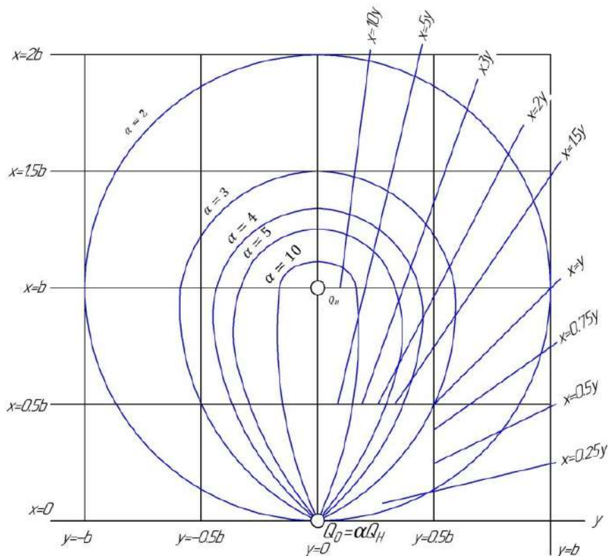
2-rasm. Debalans \alpha qiymatlarida ikki quduqli yuboruvchi quduqdan so'ruvchi skvajinagacha bo'lgan eritma aylanish maydon chegaralari
