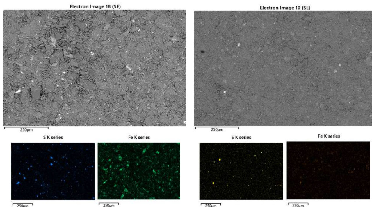
Рис. 3. ЭДС-СЭМ-анализ хвостов флотации: а – с УЗО; б – без УЗО
