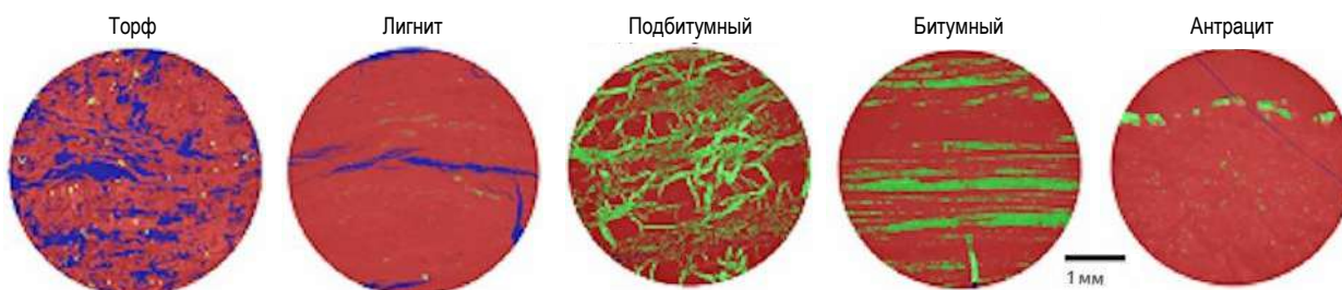
Рис. 4. Сегментированные 2D-срезы: уголь (красный), минералы (зеленый), поры/трещины (синий)
