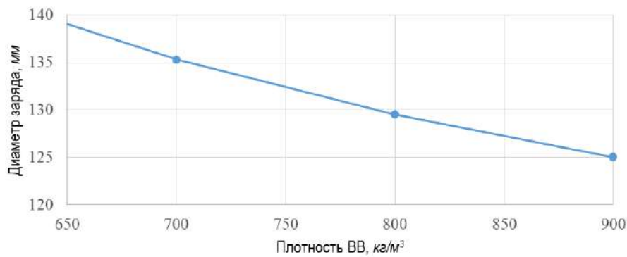
Рис. 1. Влияние плотности ВВ на изменение диаметра контурного заряда
