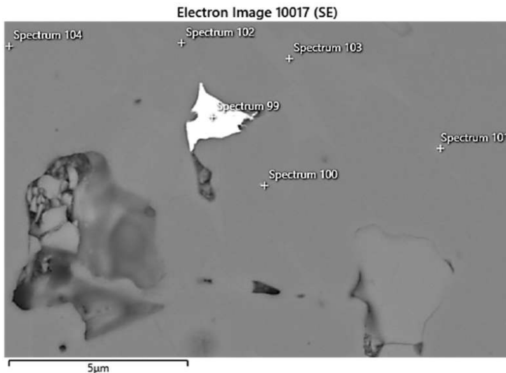
Рис. 3. РЭМ-изображение частицы золота (яркая область, Спектр 99) размером 1,7 мкм в пирите
