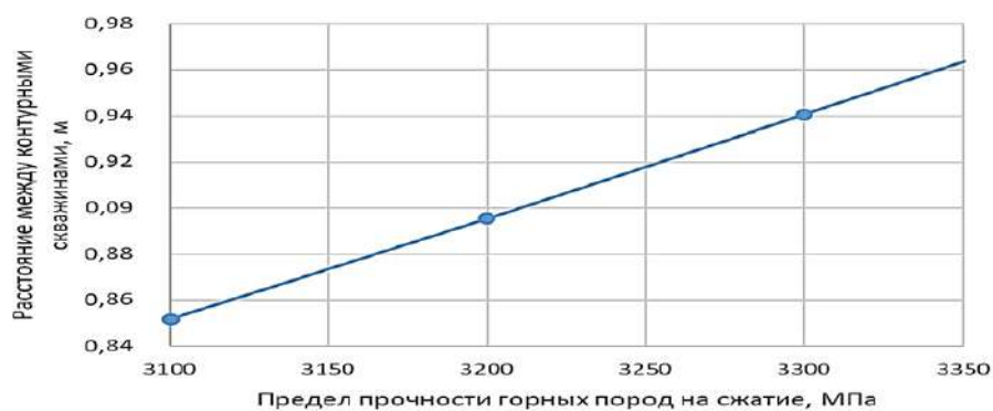
Рис. 15. Влияние предела прочности горных пород на сжатие на изменение расстояния между контурными скважинами
