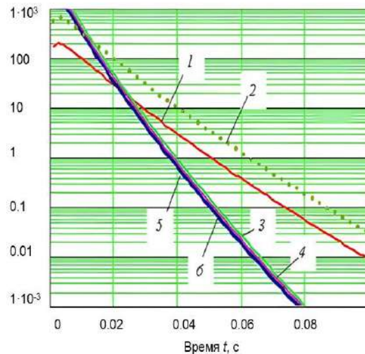
Рис. 2. Изменение скоростей смещения при разрушении породы скважинным зарядом с пеногелевой забойкой: а – общий вид; б – по логарифмической шкале; 1 – в породе; 2 – в забойке из буровой мелочи; 3, 4, 5, 6 – в пеногелевой забойке в зависимости от её плотности
