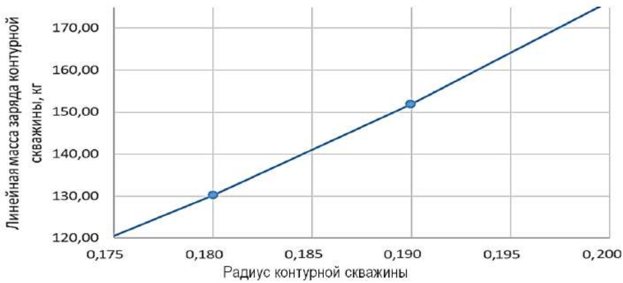
Рис. 11. Влияние радиуса контурной скважины на изменение линейной массы контурного заряда
