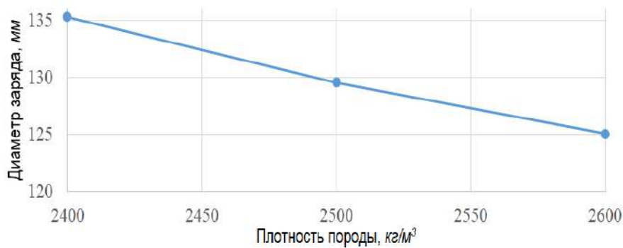
Рис. 2. Зависимость диаметра контурного заряда от плотности горных пород
