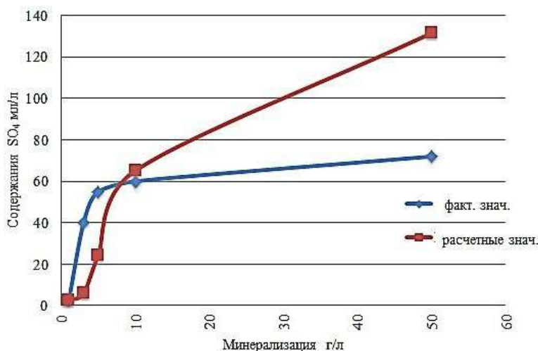
Рис. 4. Зависимость содержания SO_4^{2-} в поверхностных водах от минерализации в водах верхней гидродинамической зоны
