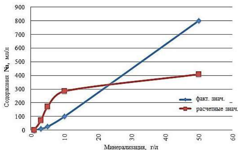
Рис. 5. Зависимость содержания Na^+ в поверхностных водах от минерализации в водах верхней гидродинамической зоны
