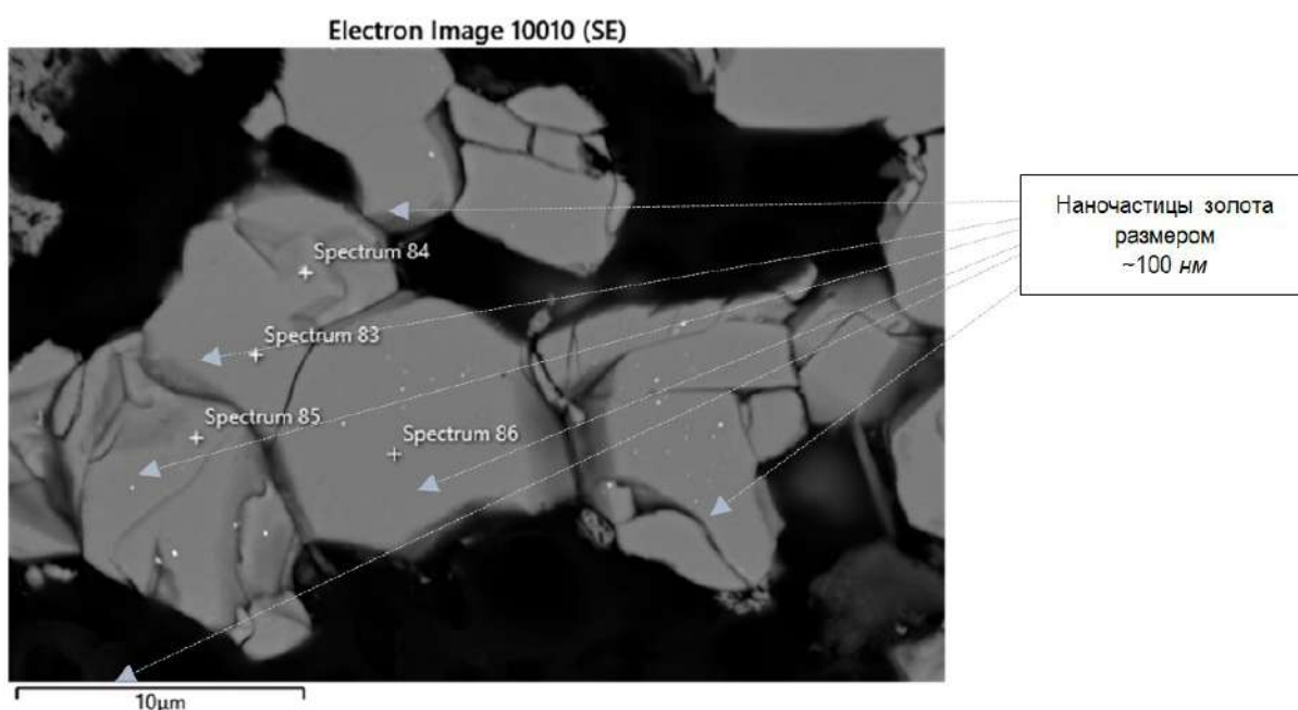
Рис. 4. Наночастицы золота в пирротине
