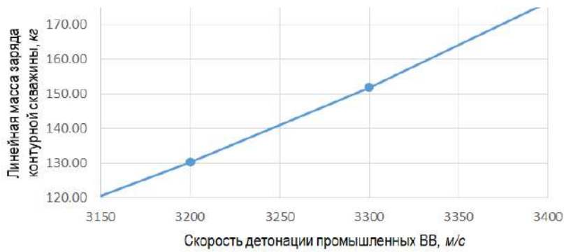
Рис. 9. Влияние скорости детонации промышленных ВВ на изменение линейной массы контурного заряда
