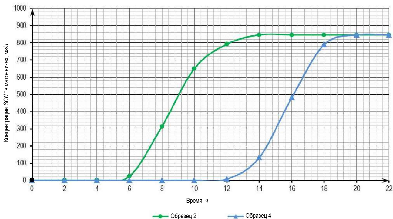
Рис. 2. График выходной кривой сорбции
