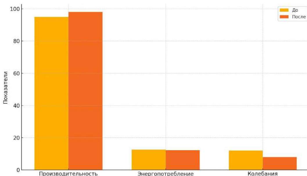
Рис. 5. Сравнение основных производственных показателей процесса измельчения руды до и после внедрения интеллектуальной системы управления на базе нечеткой логики.
