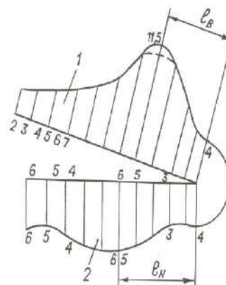
Рис. 3. Эпюры сжимающих напряжений t_{max} от воздействия на модель почвы почвоуглубительной лапы при горизонтальном усилии 20 Н: 1 – на рабочей поверхности; 2 – на нижней грани
