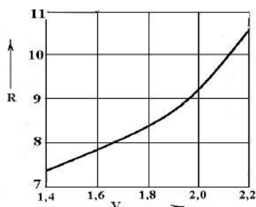
Рис. 3. Тяговое сопротивление одной пары корпусов двухъярусного плуга в зависимости от скорости движения агрегата
