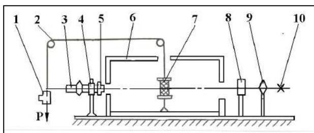
Рис. 1. Схема установки для определения оптико-механических свойств оптически чувствительных материалов
