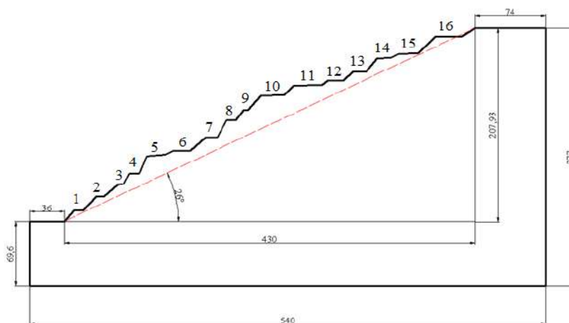
Рис. 1. Расчетная схема и габаритные размеры сечения борта
