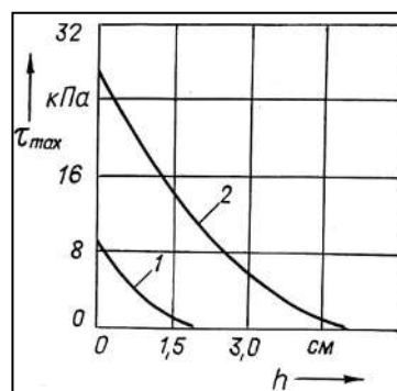
Рис. 4. Изменения t_{max} по глубине переуплотненной подшвы: 1 – для ножа-рыхлителя, 2 – для почвоуглубительной лапы
