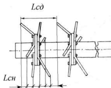
Рис. 1. Расчетная схема к определению параметров ножа с эквидистантной траекторией движения
