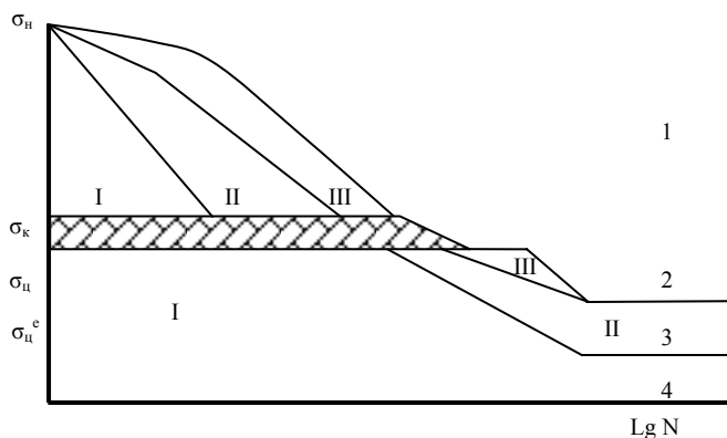
Рис. 1. Диаграмма усталостного разрушения: 1 – область малоциклового усталости (I, II и III – периоды усталости); 2 – переходная область; 3 – область многоциклового усталости; 4 – область безопасных повреждений
