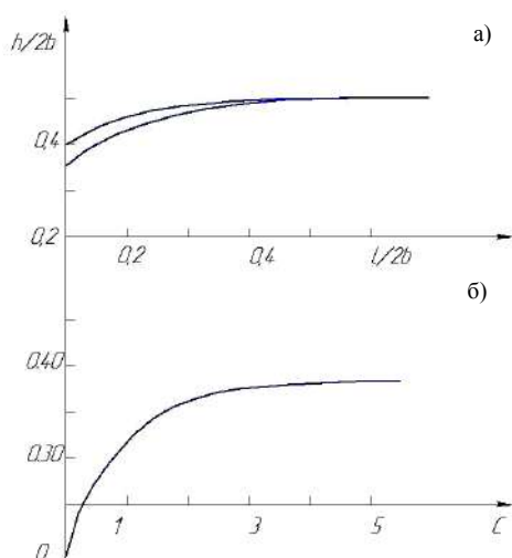
Рис. 2. Графики зависимостей: а – изменение глубины возникновения \tau_{\max} и расстояние i области циклоиды; б – изменение интервала H в зависимости от радиуса циклоиды
