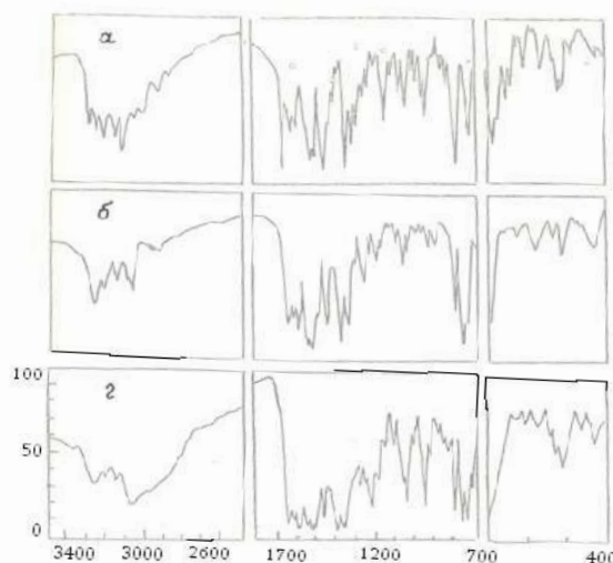
Рис. 2. Ик спектры H_2L (а), Ni(H_2L)_2 (б), Ni(HL)_2
