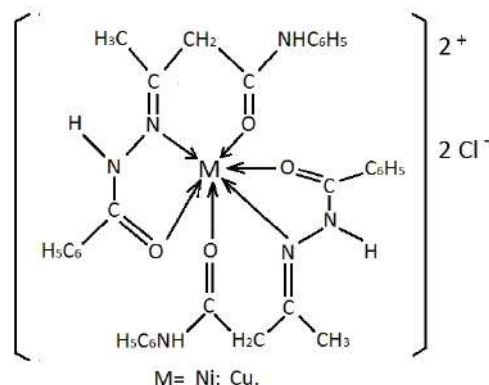
Рис. 3. Октаэдрическое строение комплекса
