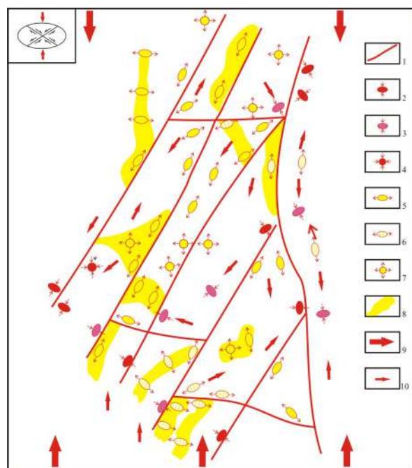
Рис. 2. Схема геодинамической обстановки периода рудообразования Даугызтауского рудного района: 1 - разломы; 2 - зона локального сжатия; 3 - предполагаемая зона локального сжатия; 4 - зона всестороннего сжатия; 5 - зона локального растяжения; 6 - предполагаемая зона локального растяжения; 7 - зона всестороннего растяжения; 8 - площади растяжений; 9 - направление региональных усилий сжатия; 10 - направление смещений
