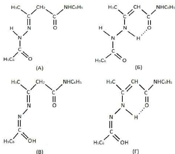
Рис. 1. Таутомерные формы лиганда
