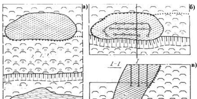
Рис. 2. Раздельное взрывание с естественным экранированием: а, б - эксплуатационный блок до и после отбойки породы со стороны висячего бока рудного тела; в - поперечный разрез блока; 1 - рудная брекчия, 2 - границы взрывных блоков, 3 - сланцы; 4 - взрывные скважины; 5 - серпентиниты
