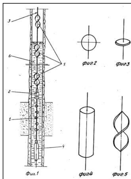
Рис. 1. Способ проведения взрывных работ в скважине
