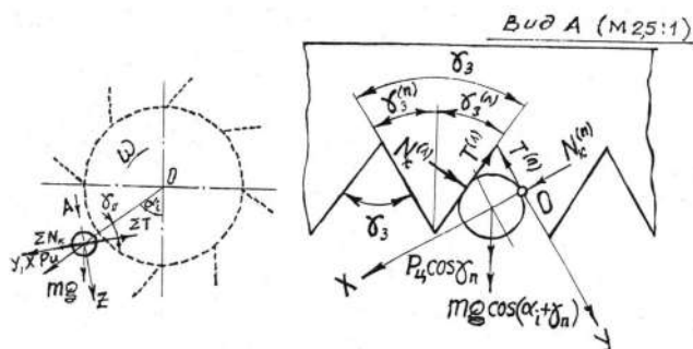
Рис. 2. Схема сил, действующих на почвенный комок, находящийся между смежными зубьями планок
