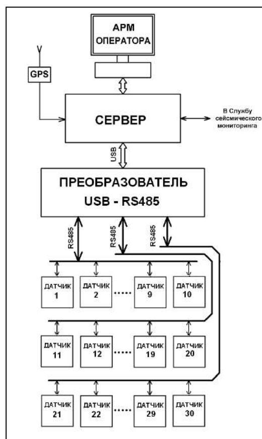
Рис. 1. Структурная схема системы мониторинга круто-наклонного конвейера КНК-270
