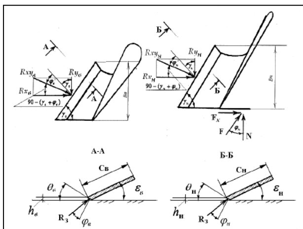
Рис.1. Схема определения тягового сопротивления верхнего и нижнего корпусов двухъярусного плуга
