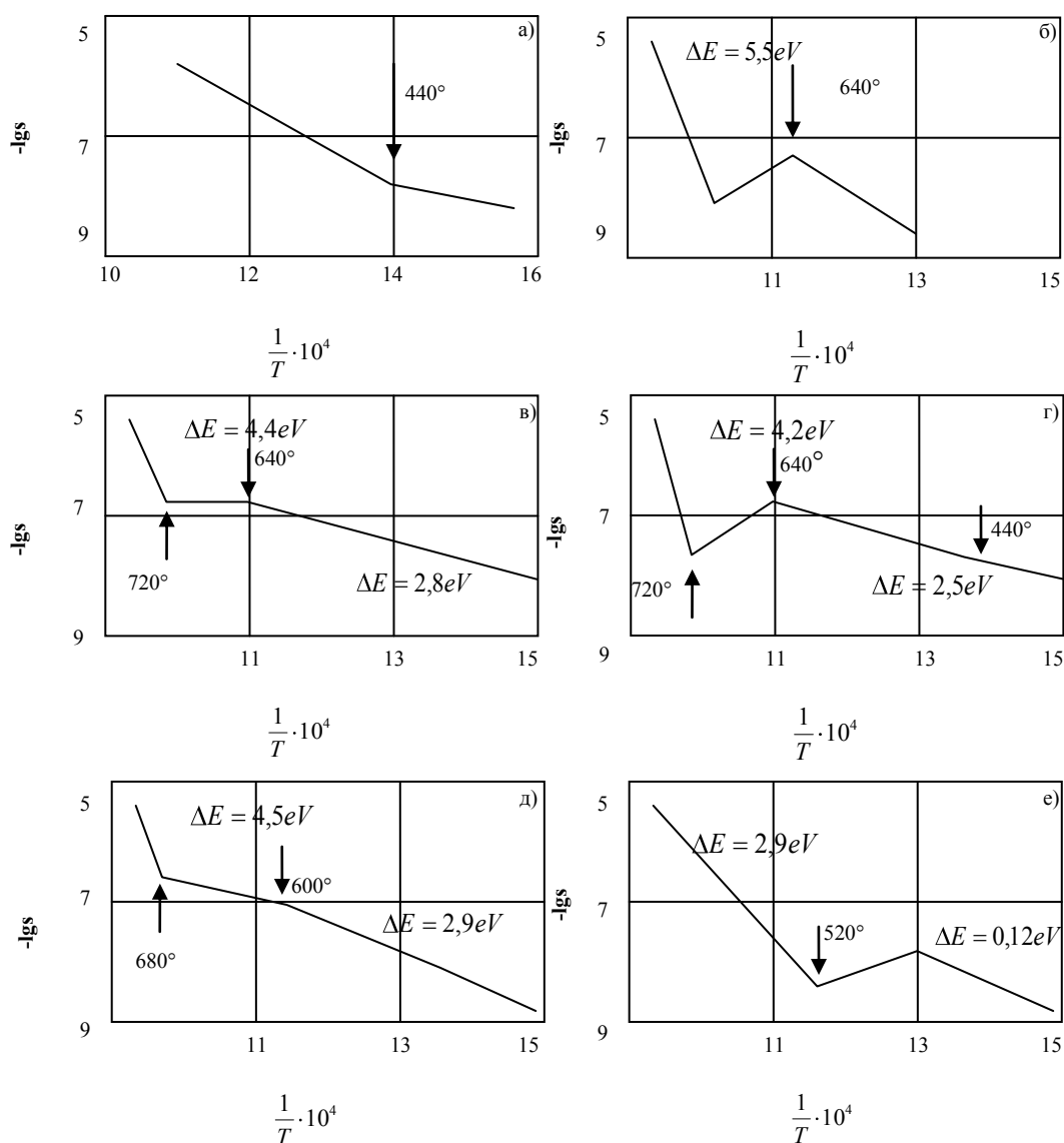
Рис. 1. Влияние температуры на электропроводность образцов из Fe_2O_3 (а), CaO (б), CaO+2Fe_2O_3 (в), 2CaO+Fe_2O_3 (г), CaO+Fe_2O_3 (д), Fe_3O_4 (е)
