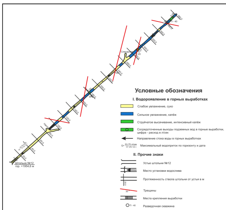
Рис. 1. Обводненность горных пород в подземных горных выработках штольни № 12 месторождения Чинарсай Хандизинского рудного поля
