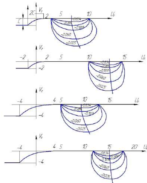
Рис. 1. Распределение напряжений в области циклоиды
