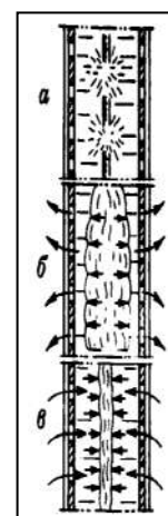
Рис. 2. Схема действия взрыва при очистке фильтра: а – тротильный шнур в момент взрыва; б – расширение газового пузыря; в – сжатие газового пузыря
