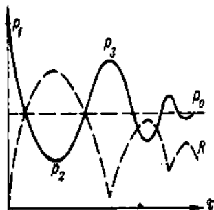
Рис. 1. Пульсация газового пузыря при взрыве заряда ВВ: p – давление в газовом пузыре; R – радиус газового пузыря; \tau – время
