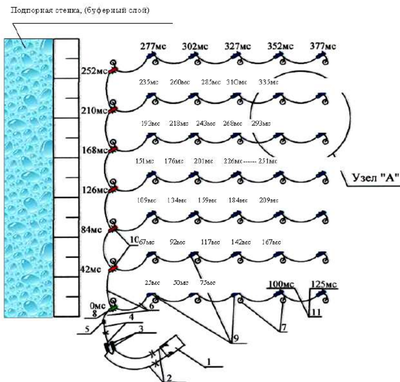
Рис. 1. Схема монтажа и последовательности инициирования скважинных взрывчатых веществ: Условные обозначения: 1 - взрывная машинка; 2 - электропровода; 3 - электродетонаторы мгновенного действия; 4 - магистральная нить детонирующего шнура; 5 - соединение детонирующего шнура с трубкой - волноводом; 6 - трубка-волновод; 7 - вертикальные скважины в плане; 8 - поверхностный соединительный блок, внутри которого находится капсуль-детонатор с замедлением 0 мс; 9 - то же, с замедлением 25 мс; 10 - то же, с замедлением 42 мс; 11 - время срабатывания поверхностных соединительных блоков без учёта прохода волны по трубкам - волноводам (мс)
