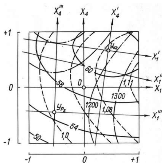
Рис. 1. Двумерное сечение поверхностей откликов, характеризующих удельное тяговое сопротивление катка, плотности и качества крошения почвы при X_2 = - 0,99 и X_3 = - 0,25 : — качество крошения почвы; - - плотность почвы; - . - . тяговое сопротивление
