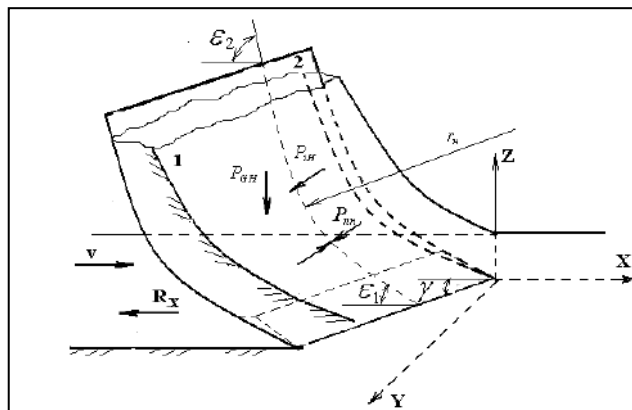
Рис. 2. Схема сил, действующих на лемешно-отвальную поверхность корпуса
