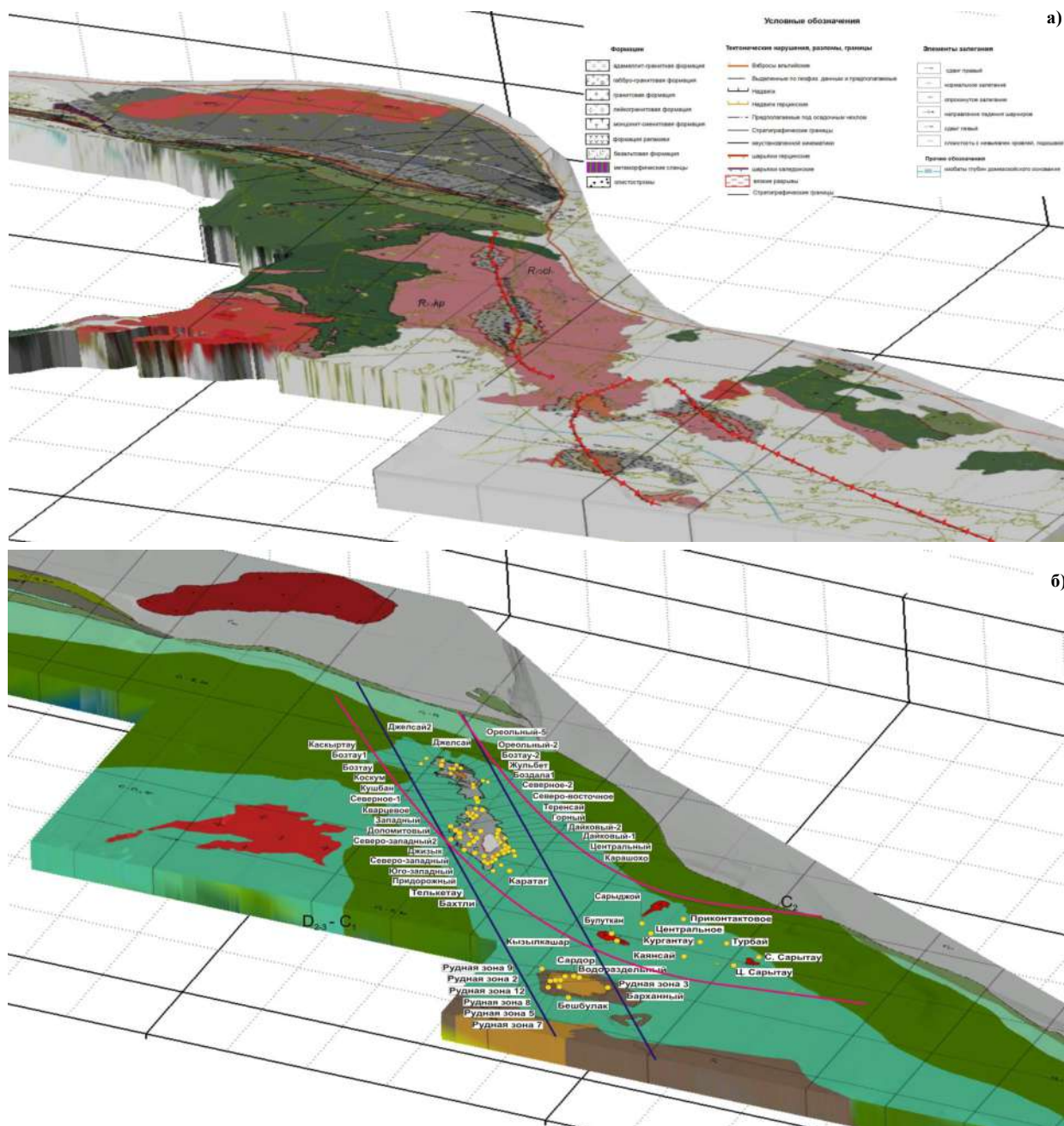
Рис. 1. Бозтау-Кокпатас-Окжетпеский тренд (БКOT) по данным геодинамических и дистанционно-съёмочных (а) и геолого-металлогенических (б) исследований
