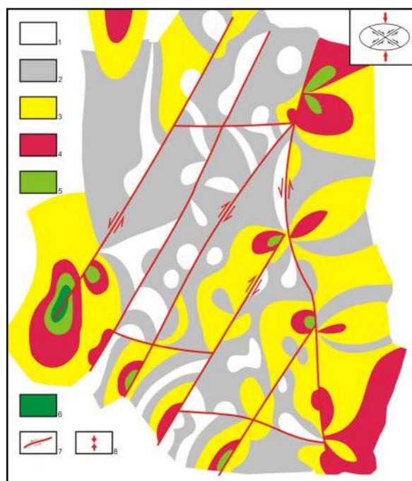
Рис. 1. Схема распределения тектонических напряжений в структурах Даугызтауского рудного района: 1 - отсутствие касательных напряжений; 2-3 - поля слабых напряжений; 4-5 - поля умеренных напряжений; 6 - поля сильных напряжений; 7 - линии разрывных нарушений и направления смещения по ним; 8 - направления активных смещающих усилий
