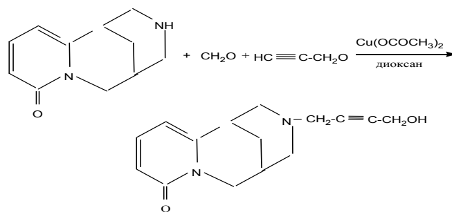
Рис. 1. Схема получения производных цитизино-бутин-2-ола-1
