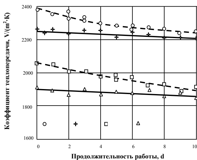
Рис. 1. Изменение коэффициента теплопередачи в зависимости от продолжительности работы аппарата: 1 и 3 – при оптимальном уровне; 2 и 4 – с развитым экономайзерным участком; 1 и 2 – вода; 3 и 4 – 60% - ный раствор роданистого аммония.
